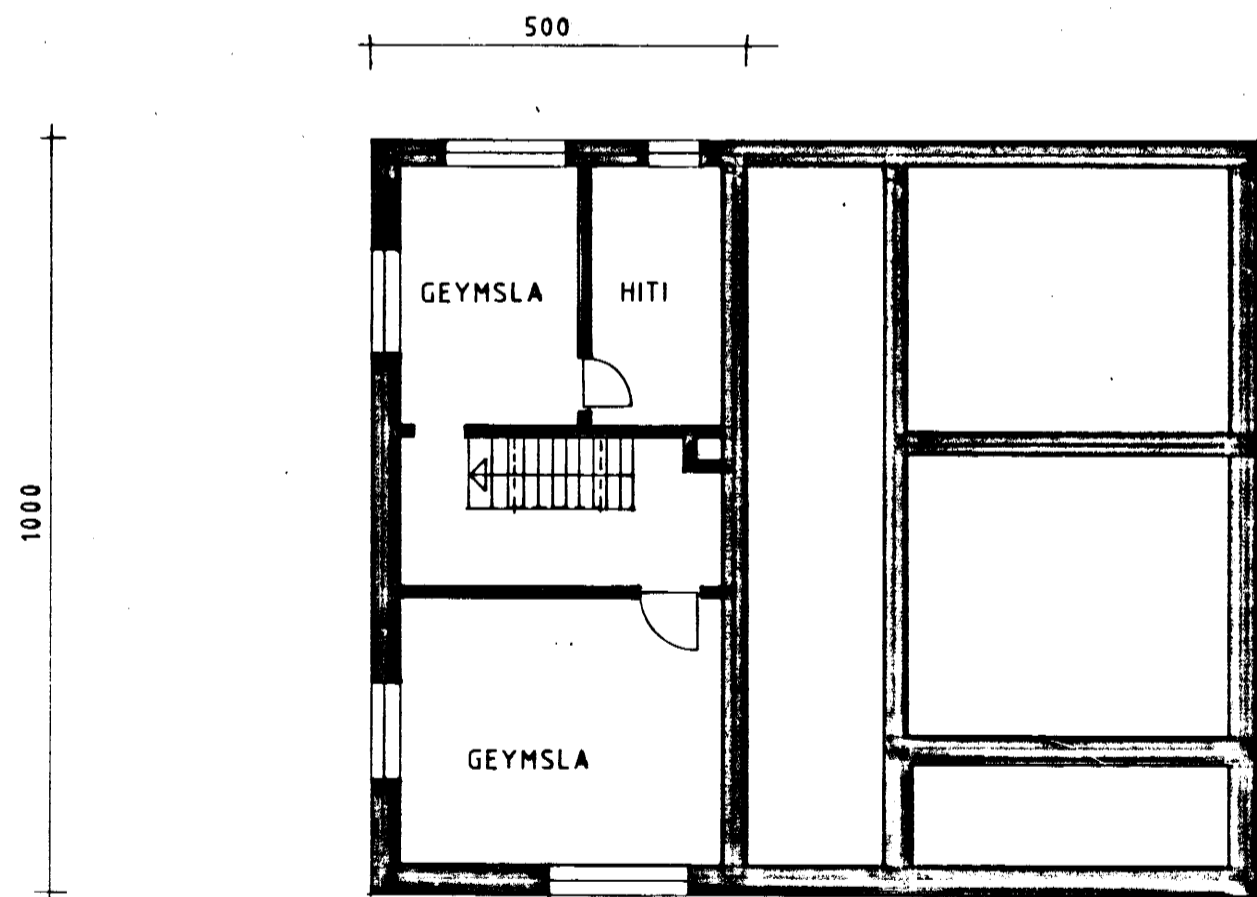
GRUNNMYND KJALLARA m.1:100
