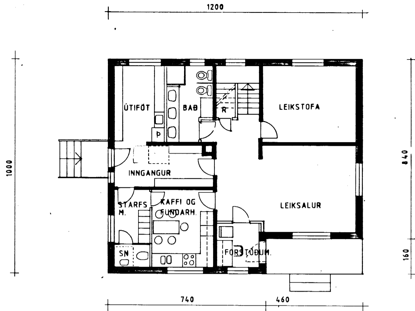
GRUNNMYND HÆÐAR m.1:100
