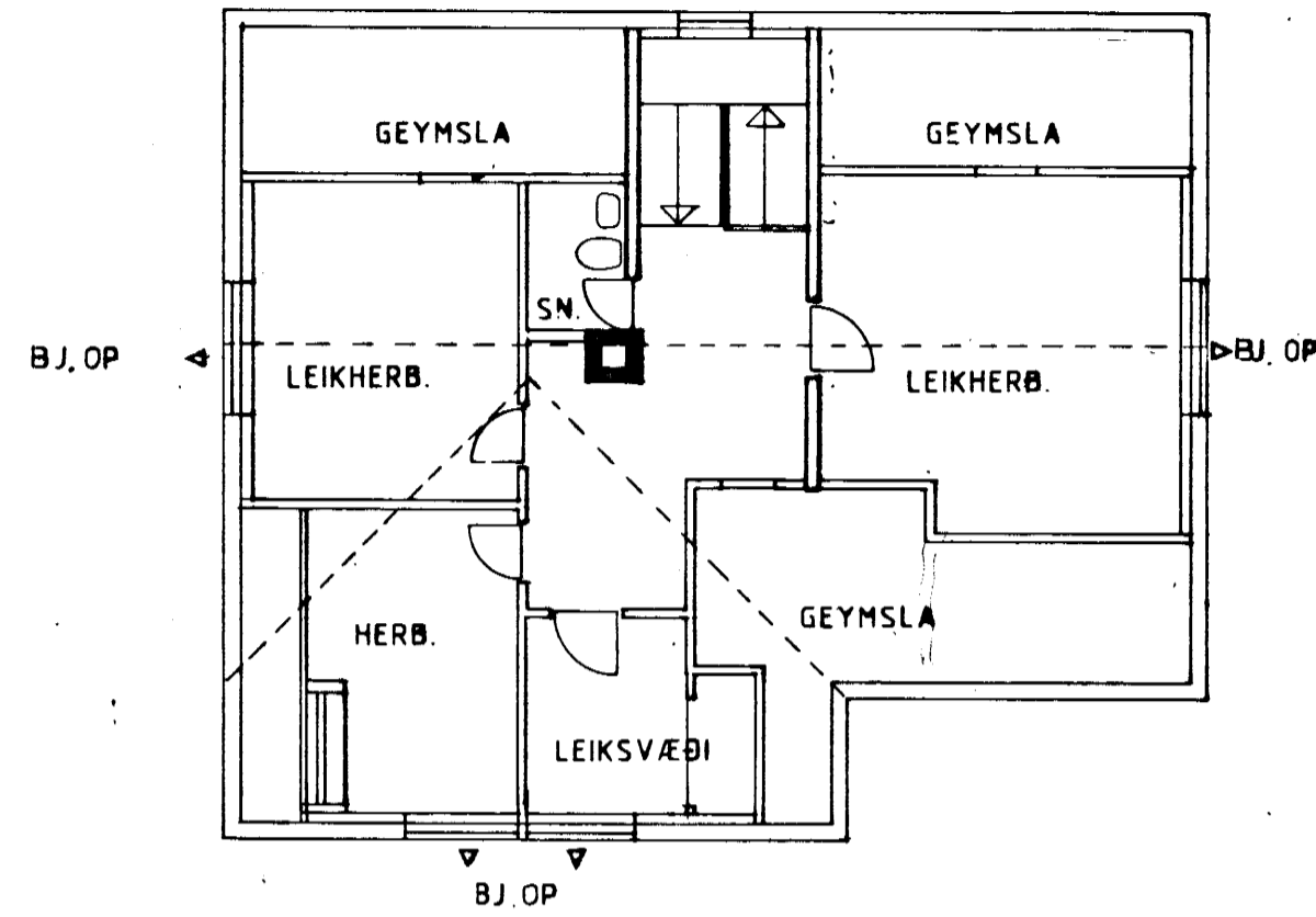
GRUNNMYND RISHÆÐAR m.1:100
