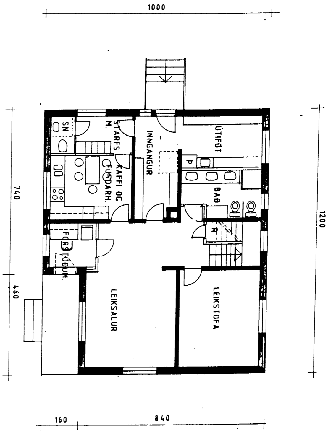
GRUNNMYND HÉÐAR m.1:100
