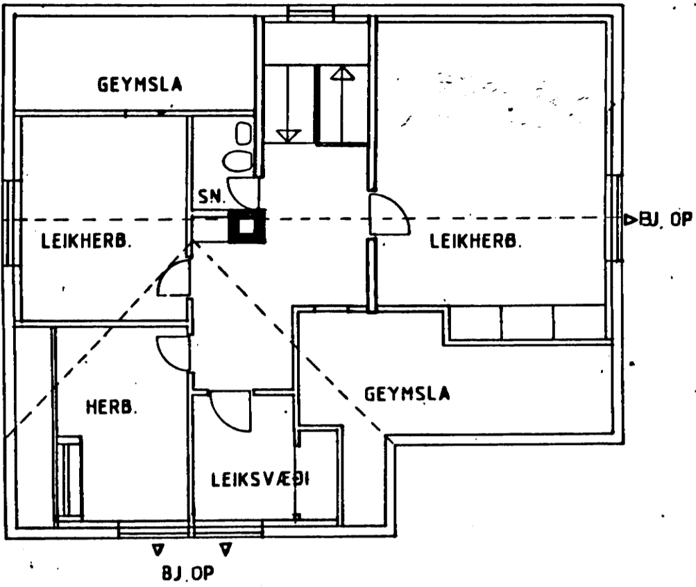
GRUNNMYND RISHÆÐAR m.1:100
