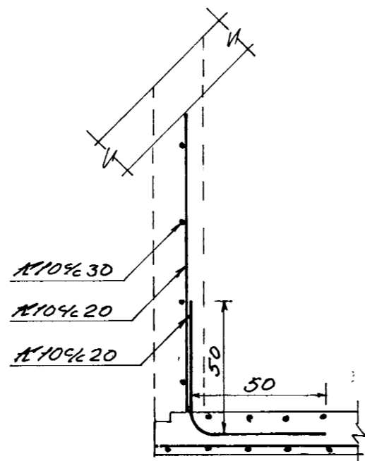
SNIA A-A 1:20
