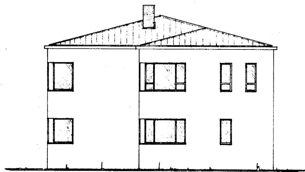
AUSTUR
