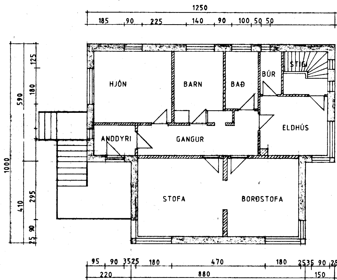
GRUNNMYND HÆÐAR 1:100
