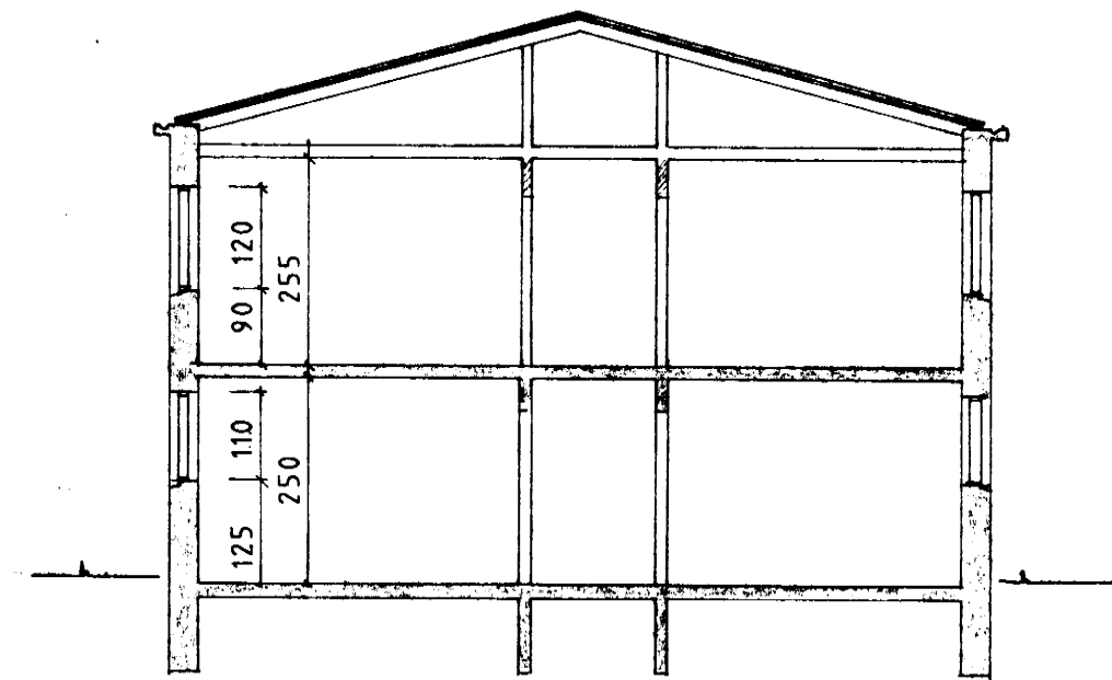
SNIB A-A 1:100
