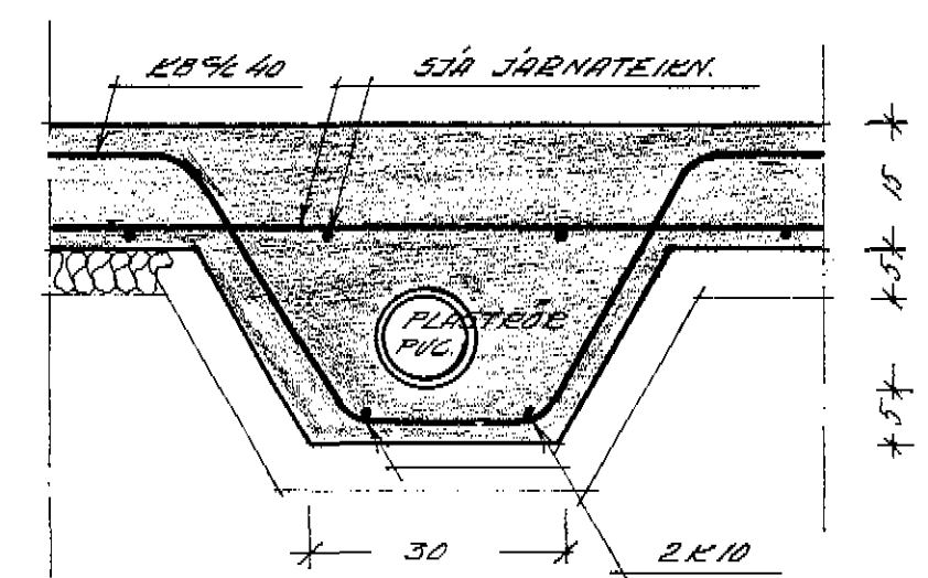
SÉRMYND I. FRÁGANGUR PLASTRÓSA Í BRUNNI ÞEGAR EKKI ER LAGT Á TITRARA FYLINGU.
