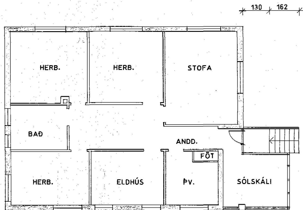
GRUNNMYND M 1:100
