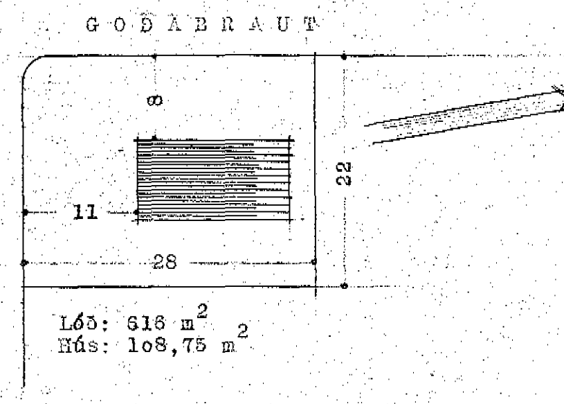
AFSTÖÐUMYND 1:500
