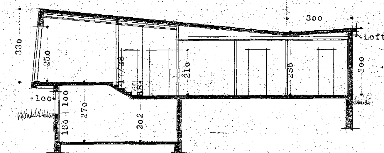
SKURÐUR
