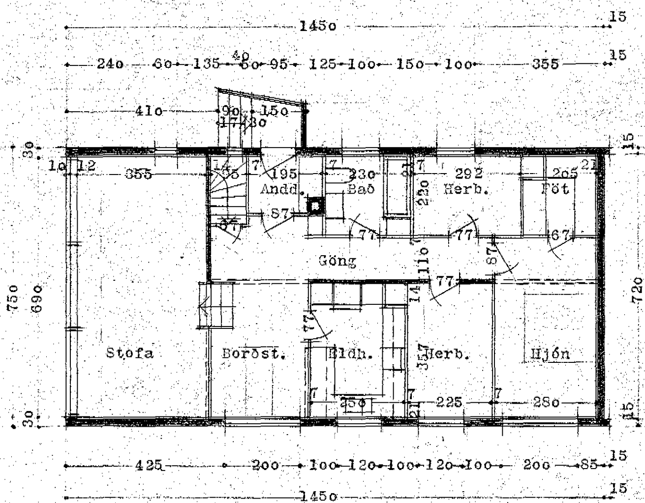
GRUNNMYND 1. HÆÐAR
