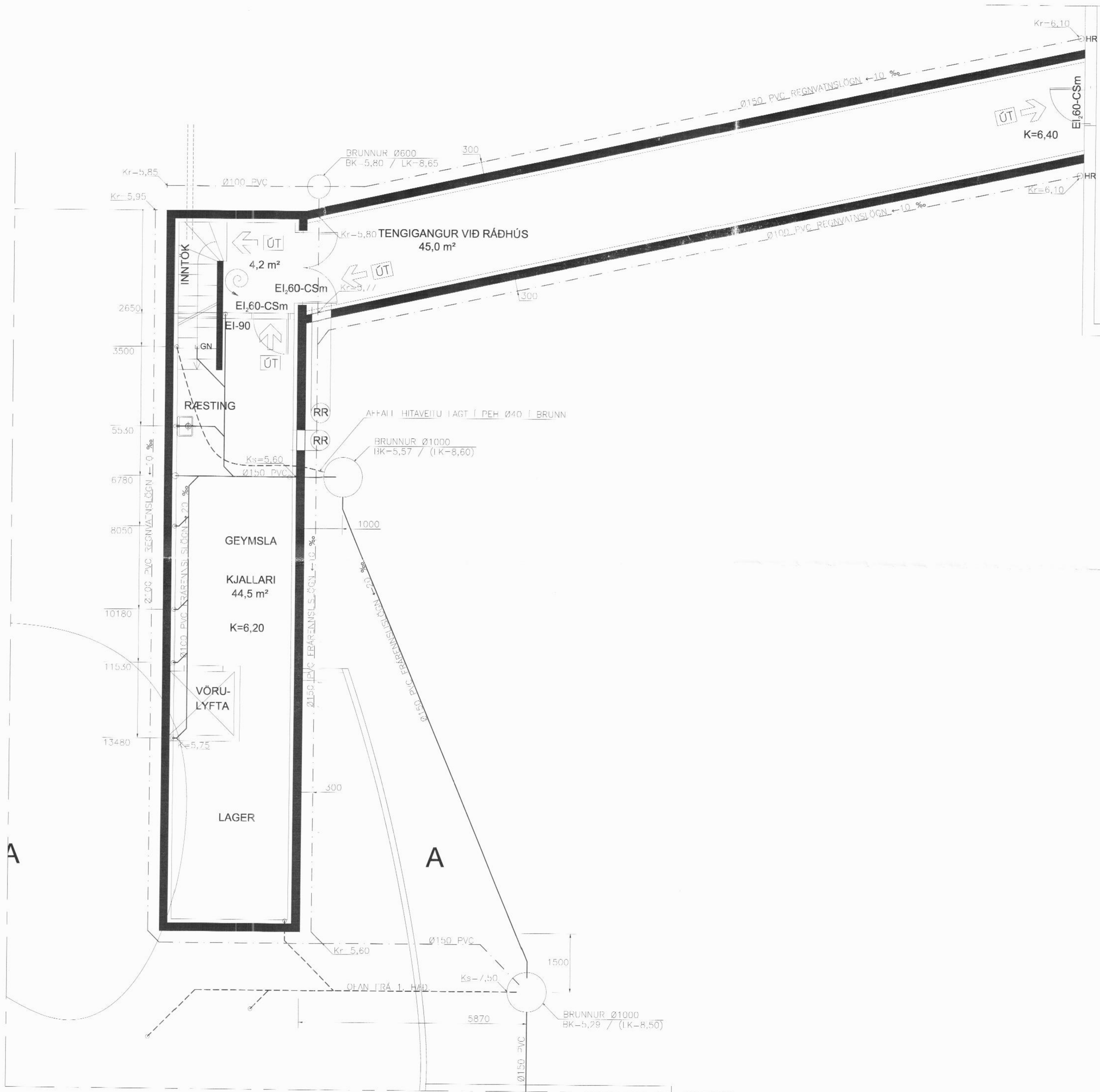
GRUNNMYND - KJALLARI, MKV. 1:50
