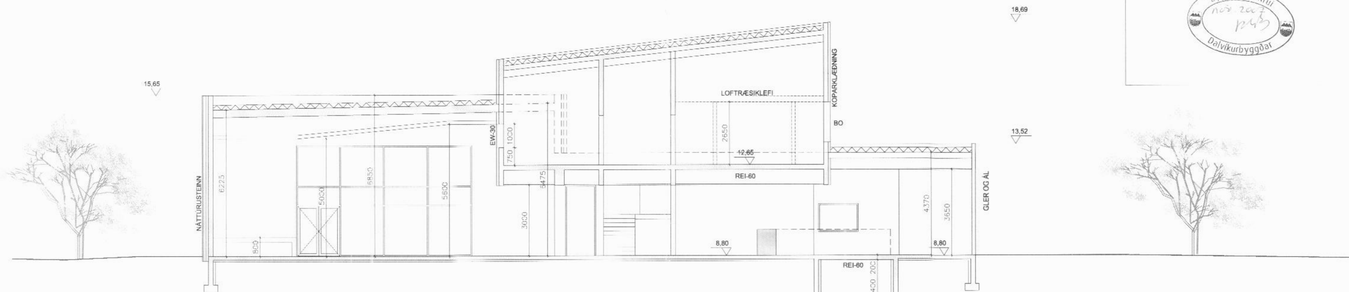
SNID A-A M 1:100 @ A2
