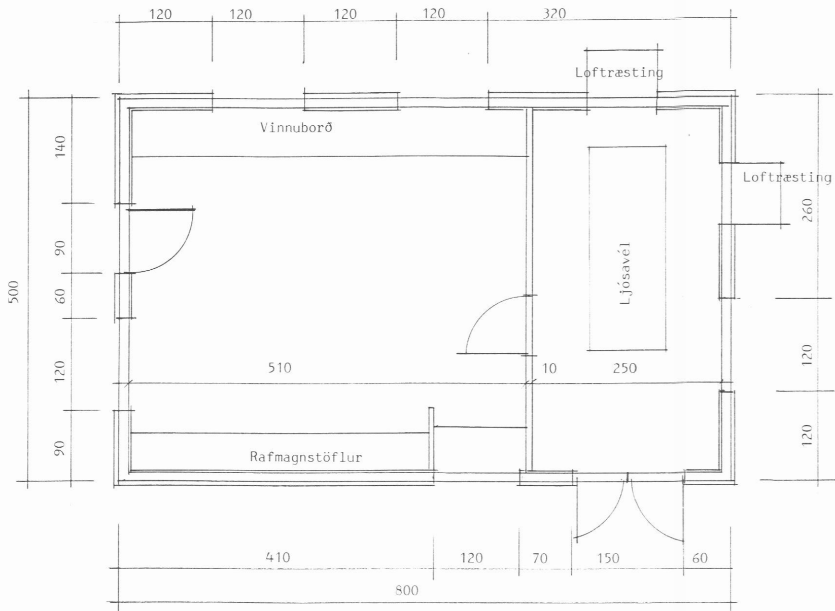
Grunnmynd
