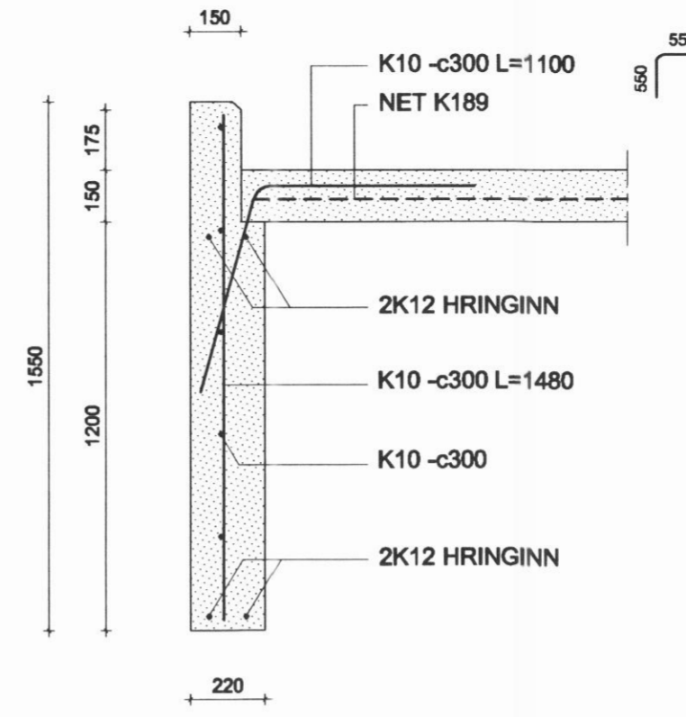
SNID 1-1 MKV. 1:20
