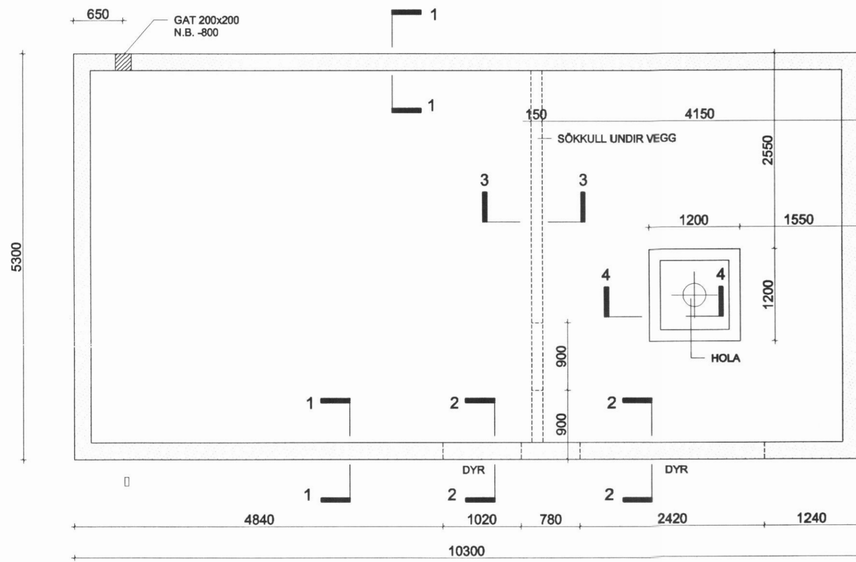
GRUNNMYND MKV. 1.50
