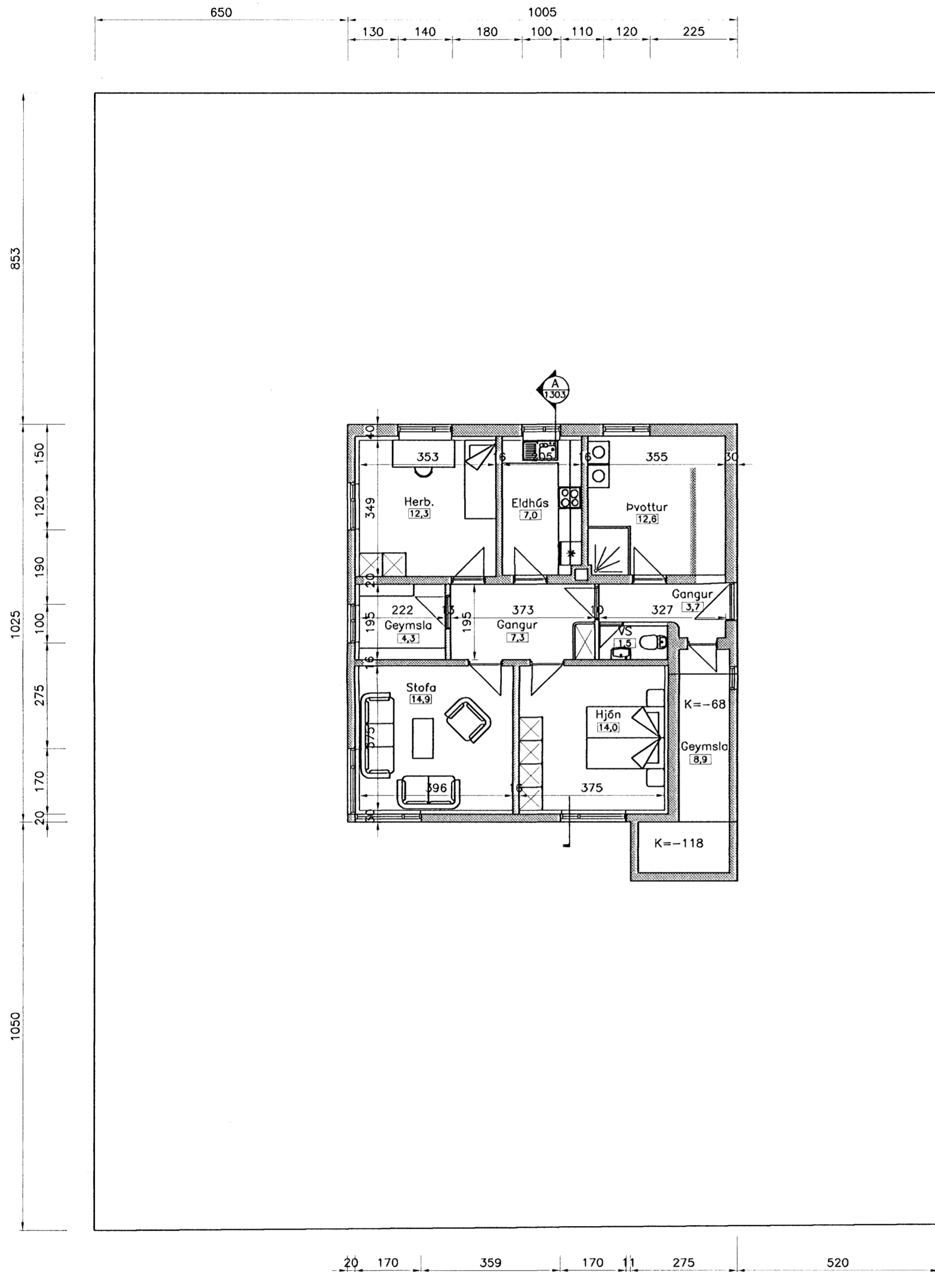
Grunnmynd 1.hæðar 1:100
