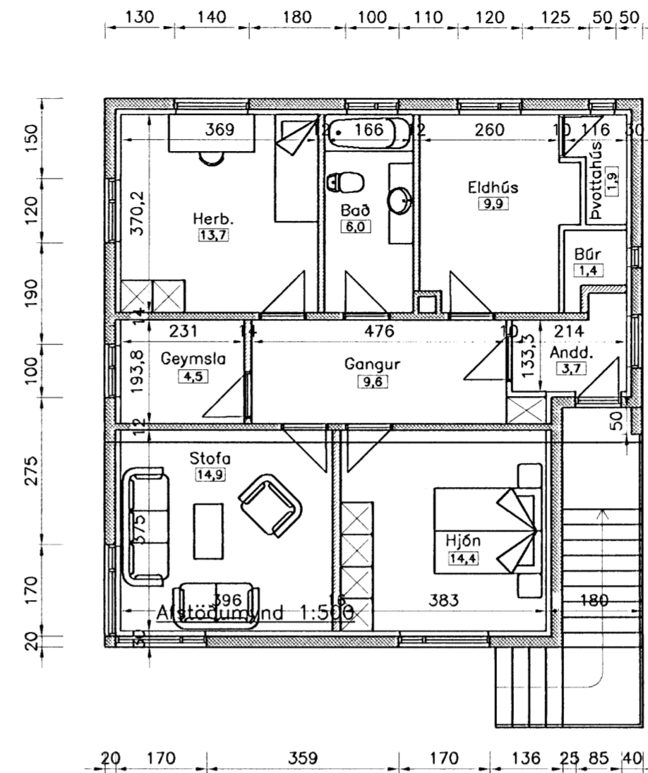
Grunnmynd 2.hæðar 1:100
