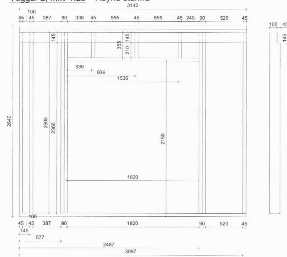
Veggur 2, mkv 1:25 Ásýnd utanfrá
