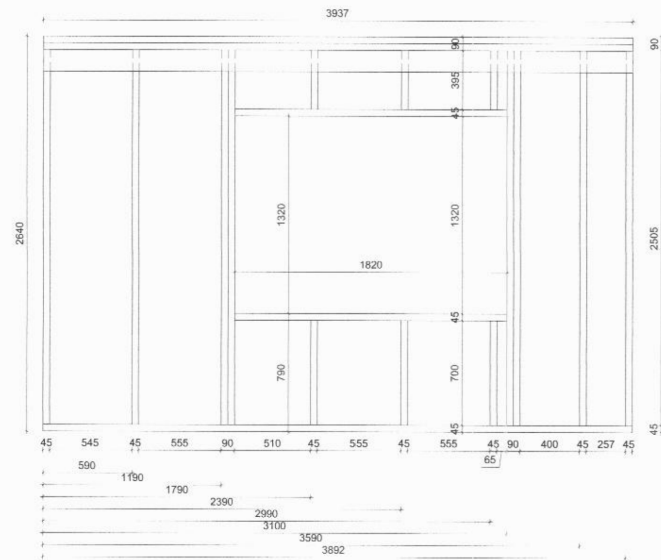
Veggur 3, mkv 1:25 Ásýnd utanfrá
