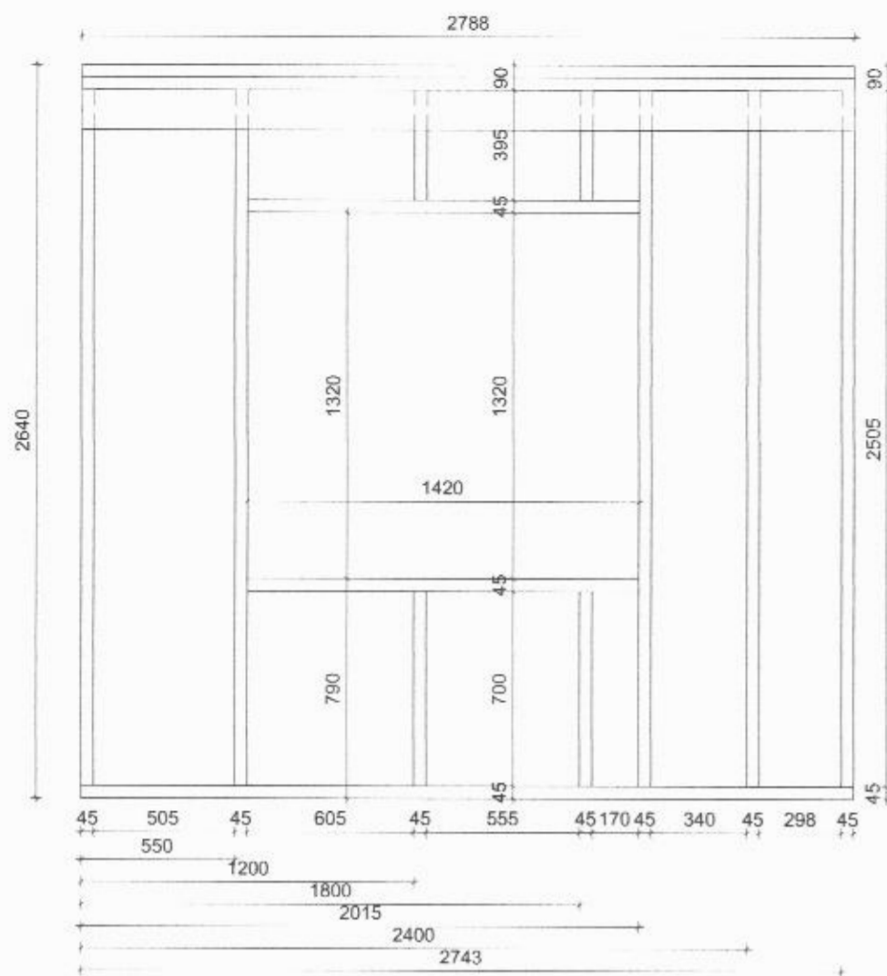
Veggur 1, mkv 1:25 Ásýnd utanfrá
