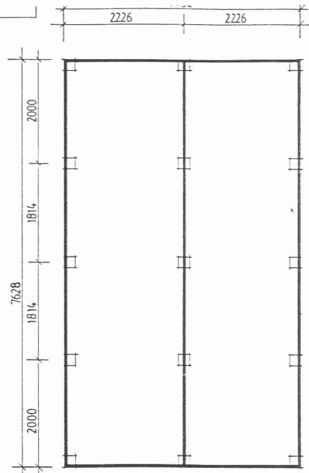
GRUNDPLAN
