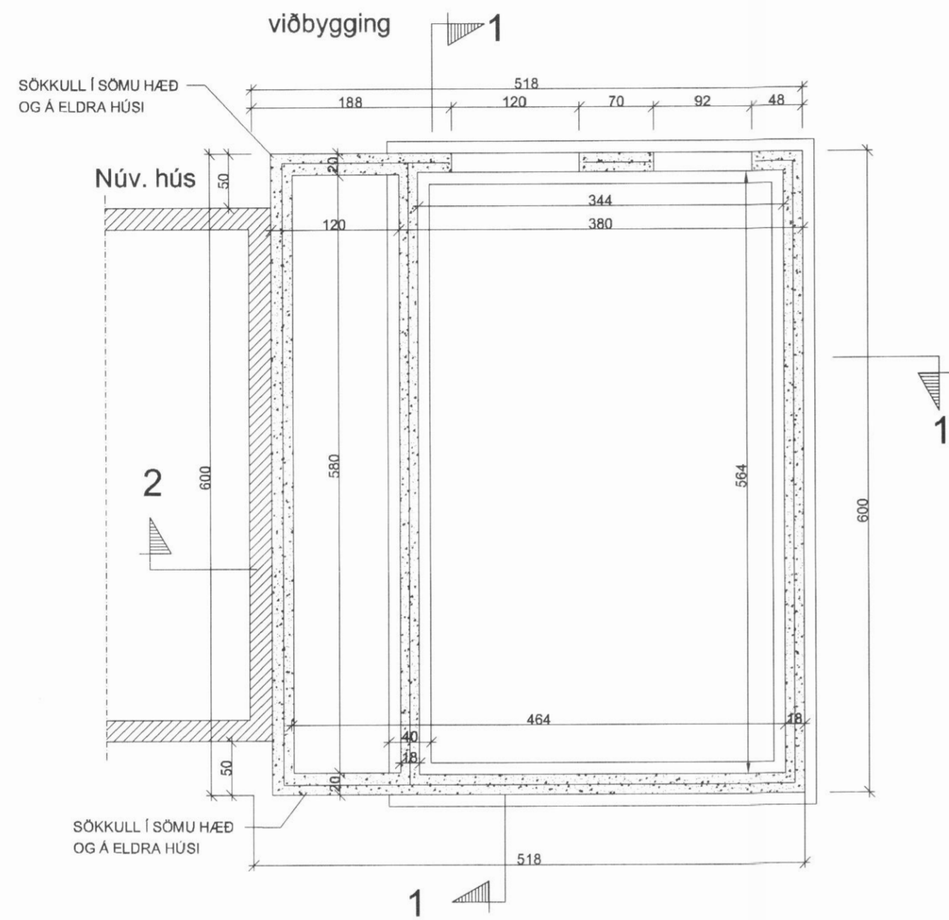
GRUNNMYND SÖKKLA KJALLARA, 1:50
