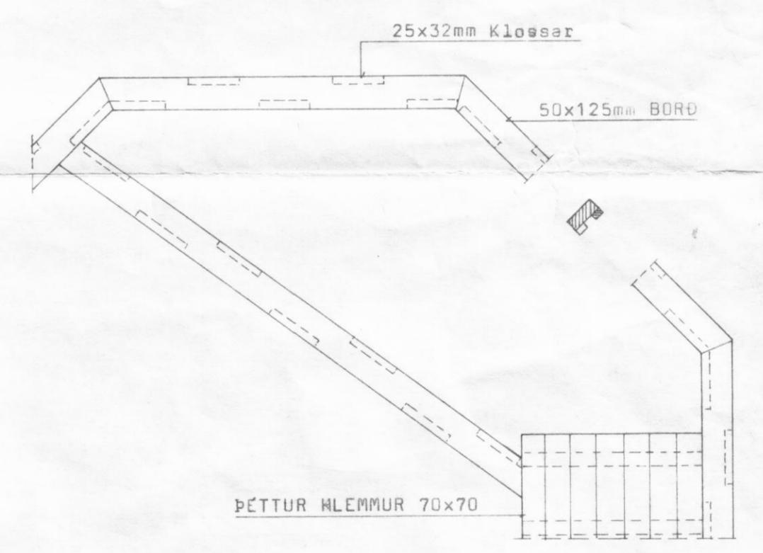
FRÁRENNSLI Á GÓLFI Í VOTHEYSTURNI M=1:20
