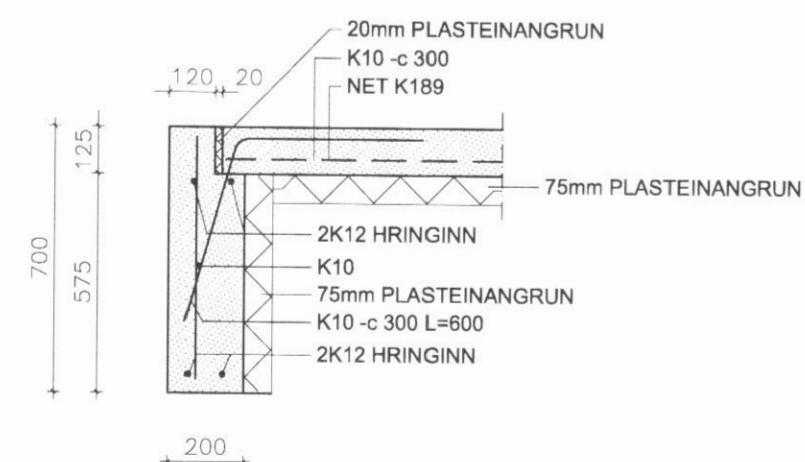
SNIÐ 1-1 MKV. 1:20
