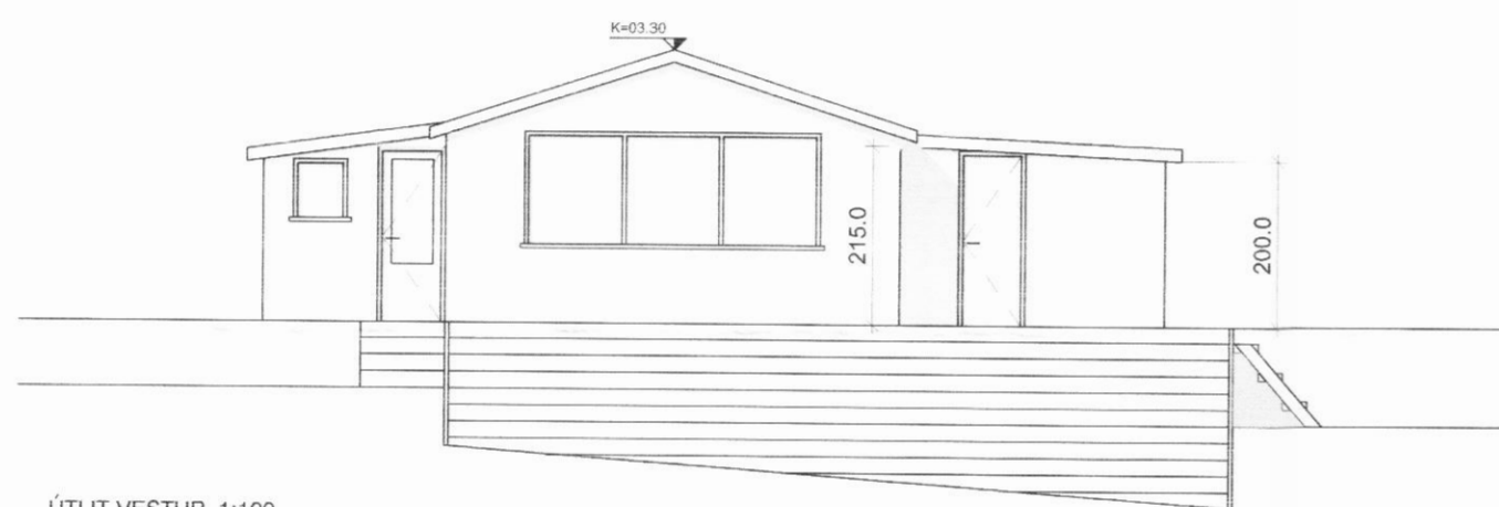
ÚTLIT VESTUR, 1:100
