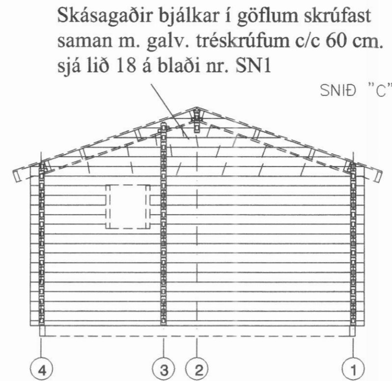
Hliðarmynd gafl festing skásagaðra bjálka
