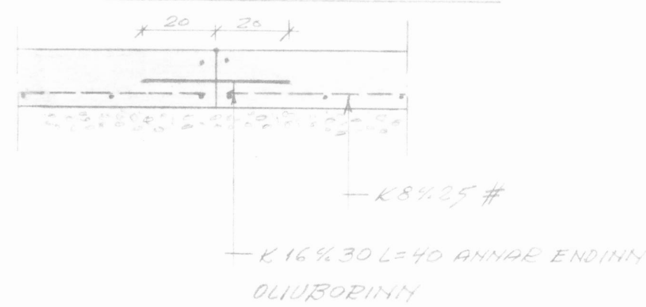
SAMSK. Á GÖLFPL. 1:10
