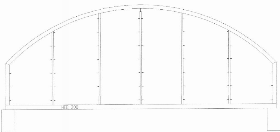
Stálgrind í norðurhlið MKV 1:100
