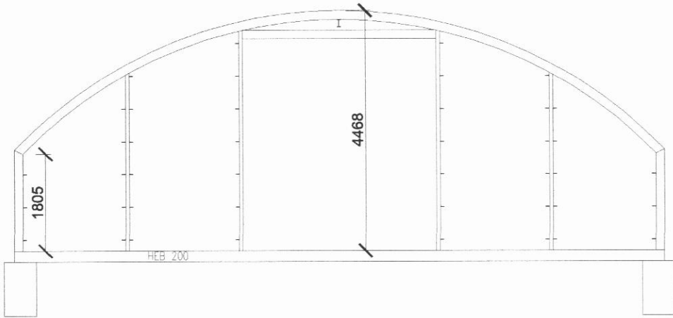
Stálgrind í suðurhlið MKV 1:100
