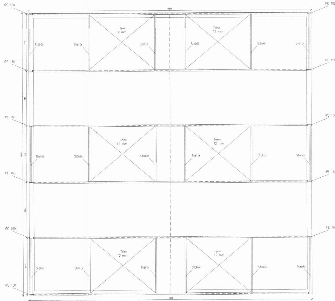
Stálgrind / Þakvirki MKV 1:100
