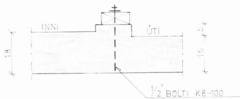
SNID A-A M=1:10
