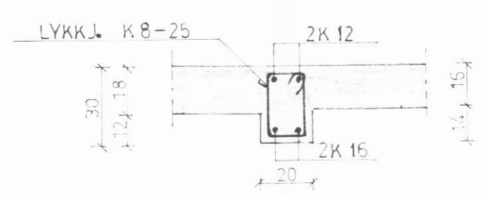
SNID í B1 M=1:20
