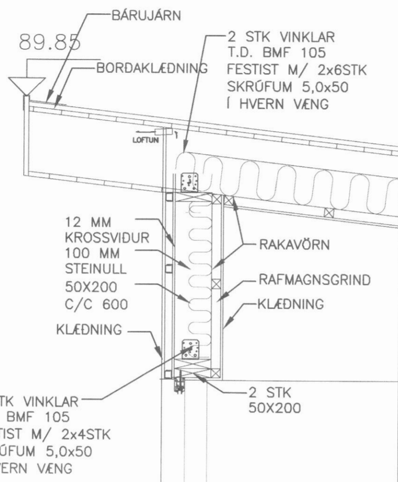
04 DEILI 08 09 1:50
