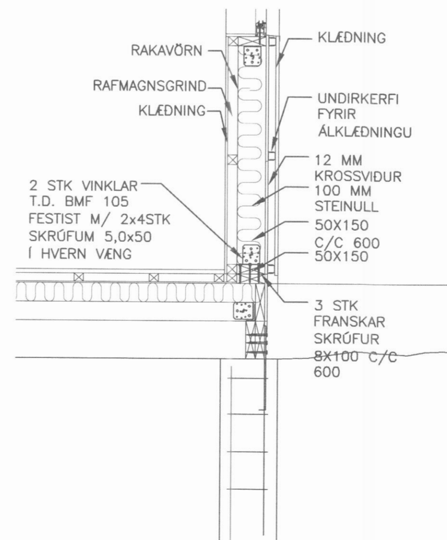
03 DEILI 08 09 1:50
