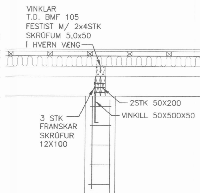
02 DEILI 08 09 1:50
