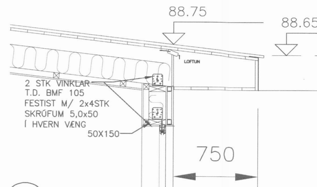
06 DEILI 08 09 1:50
