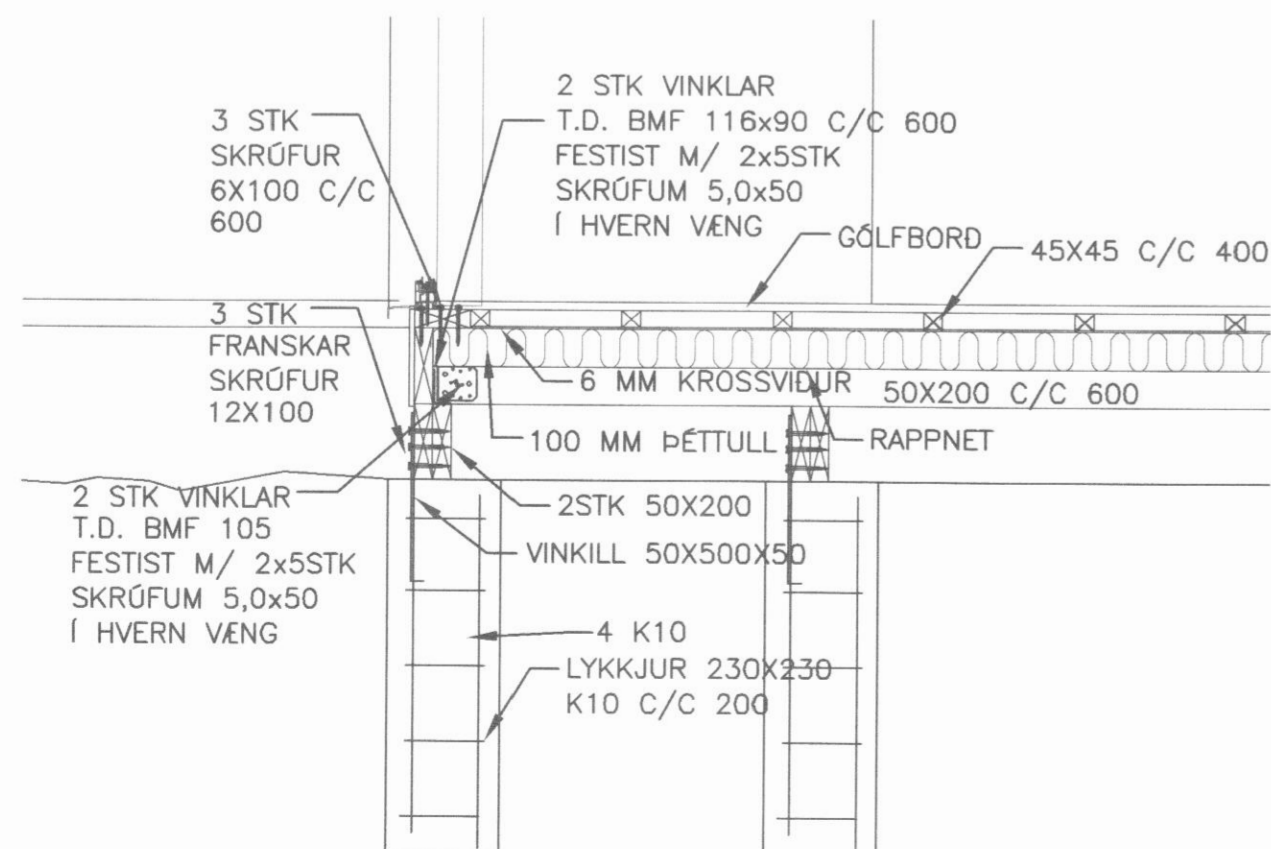
01 DEILI 08 09 1:50
