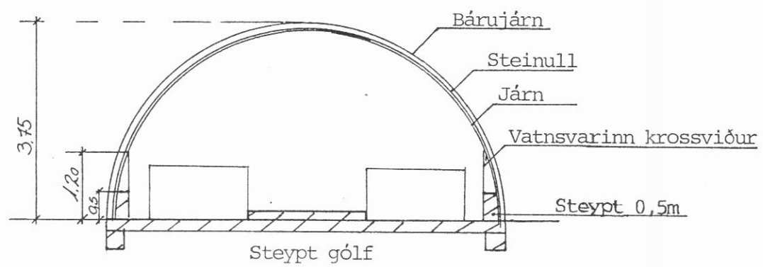
Snið A
