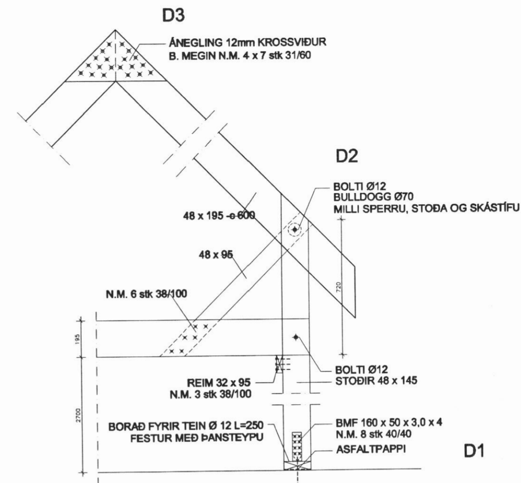
DEILI MKV.1:20
