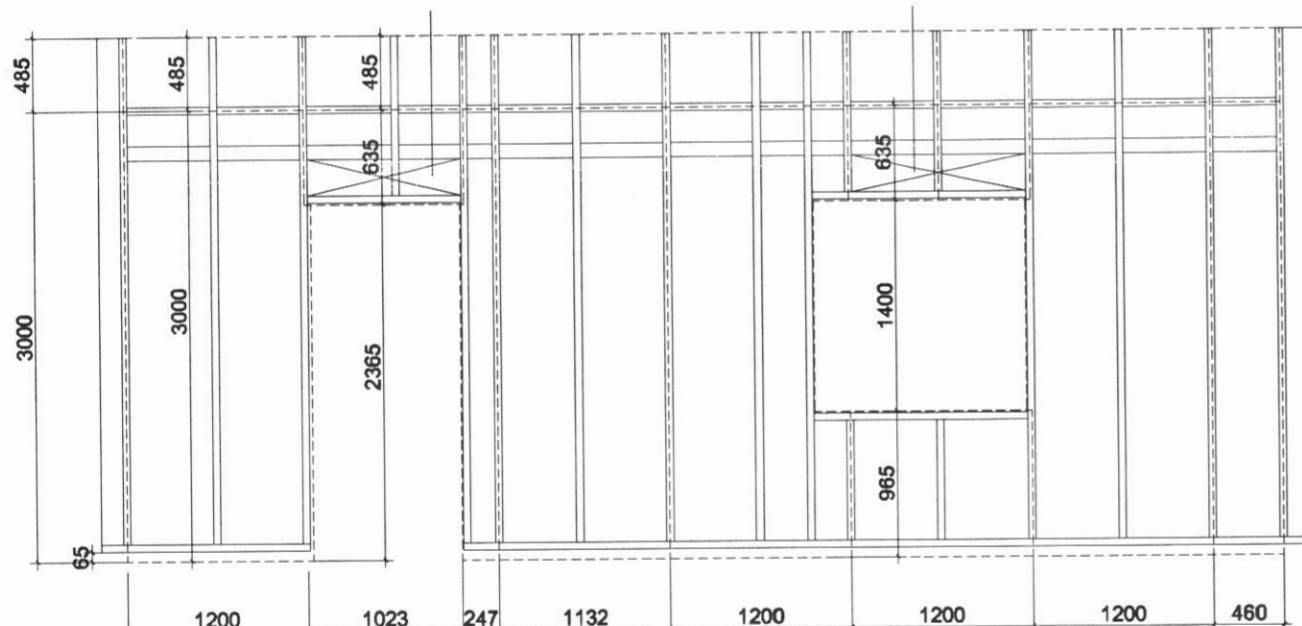
GRINDUR V05 MKV.1:50
