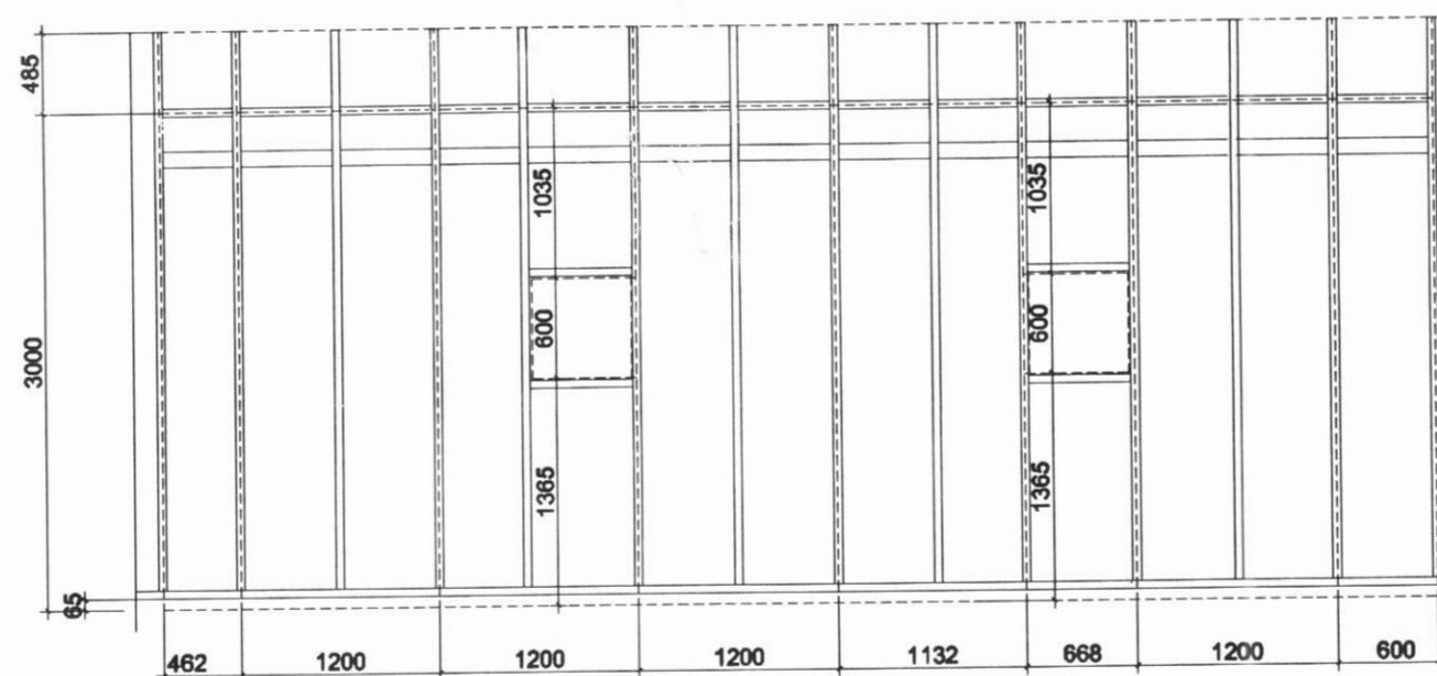
GRINDUR V06 MKV.1:50
