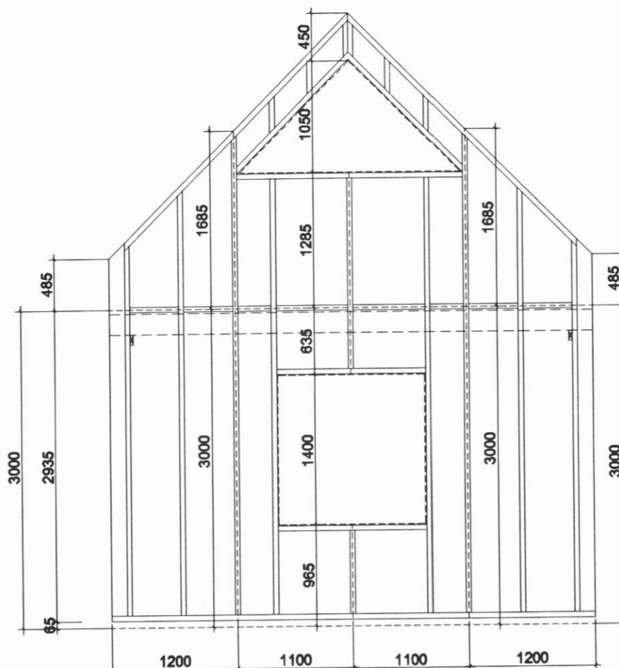
GRINDUR V08 MKV.1:50
