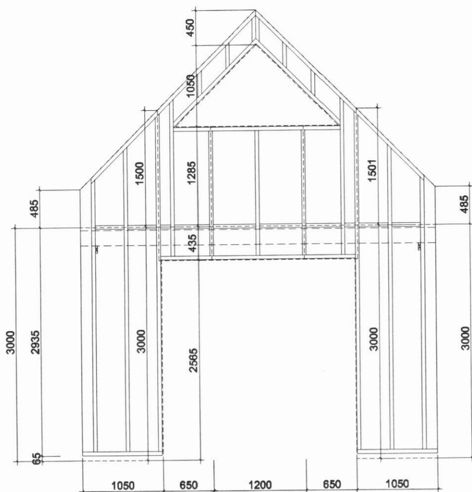
GRINDUR V07 MKV.1:50
