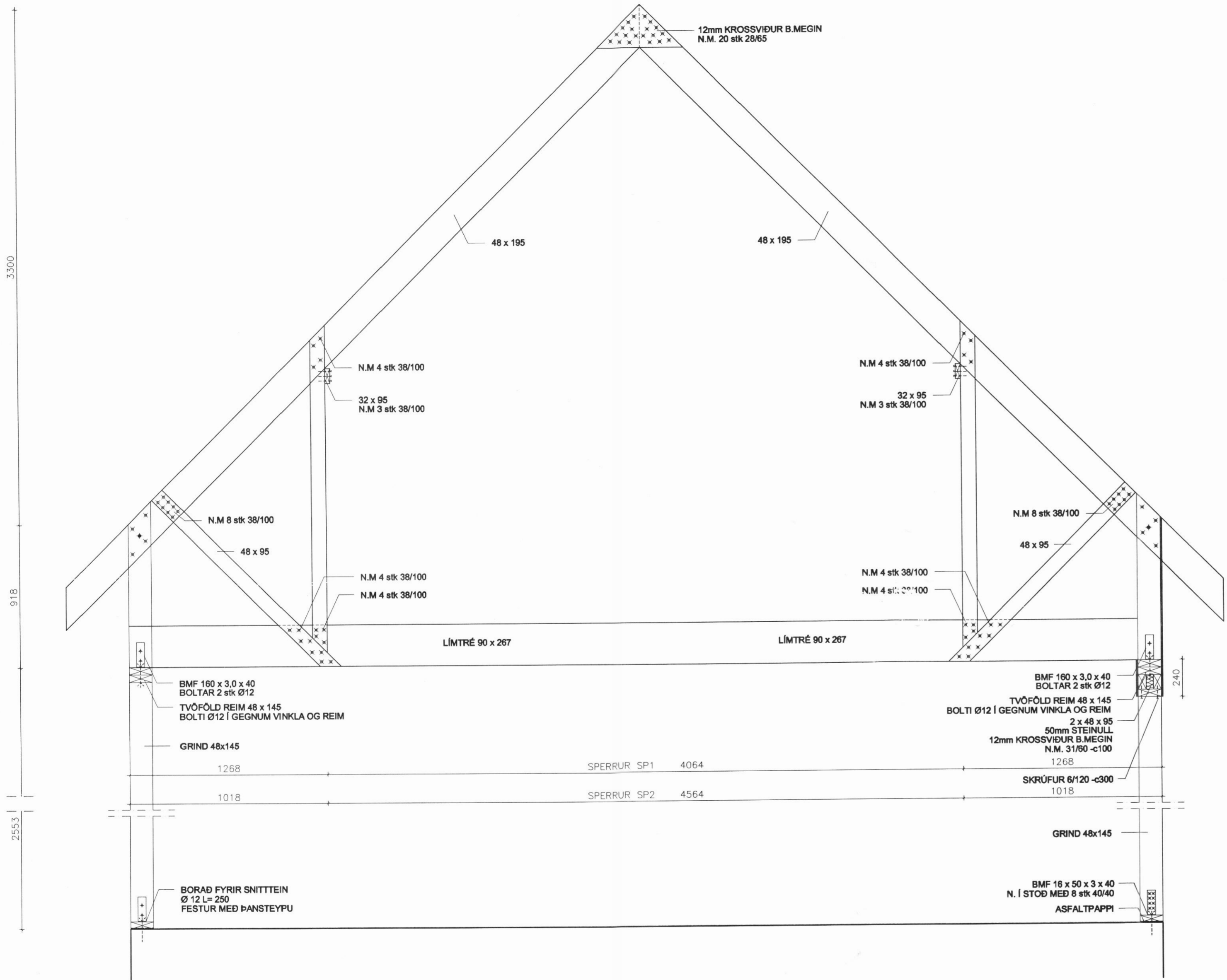
SP2 SNIÐ 2-2 MKV.1:20
