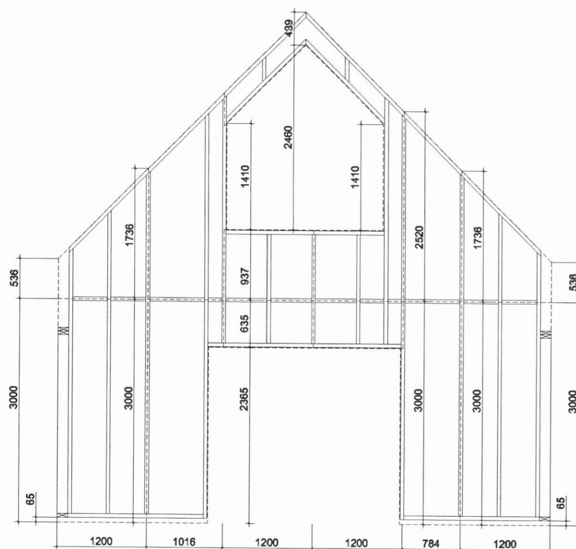
GRINDUR V03 MKV.1:50
