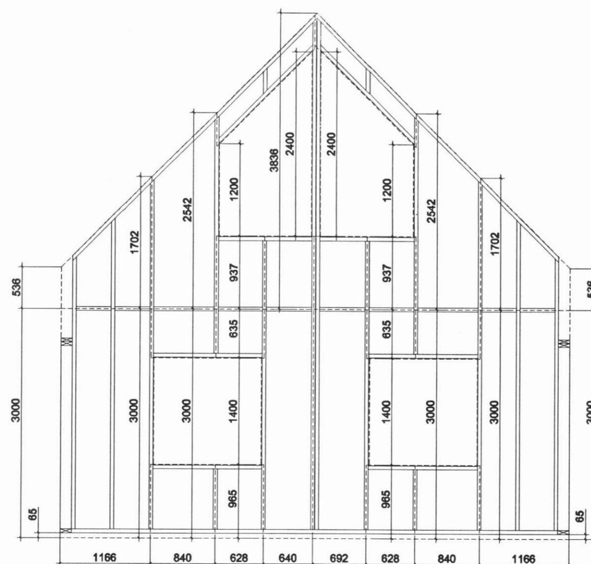
GRINDUR V04 MKV.1:50
