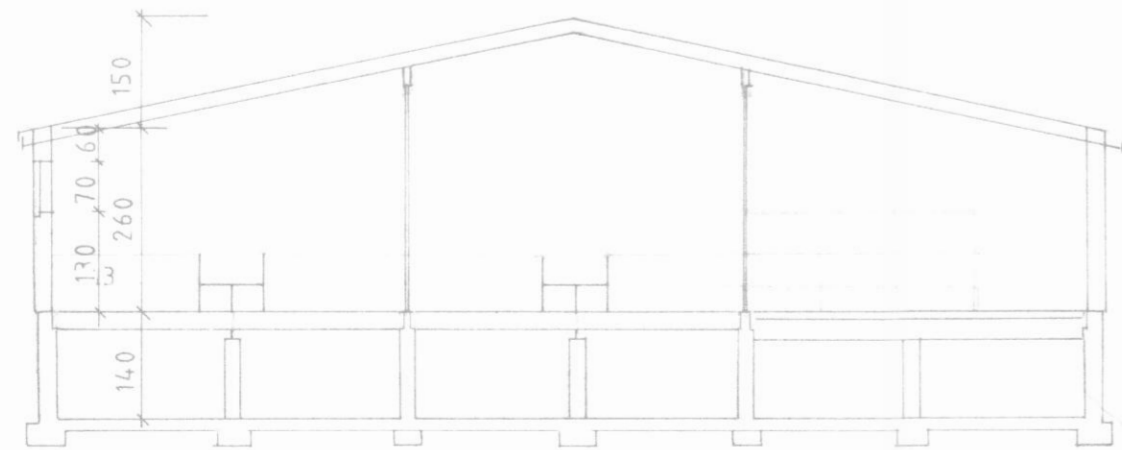
SNEIDING A - A 1:100
