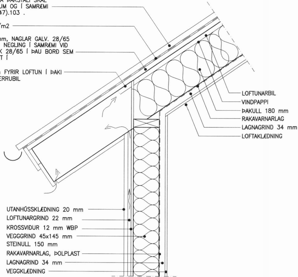
FRÁGANGUR VIÐ ÚTVEGG OG ÞAK 1:10
