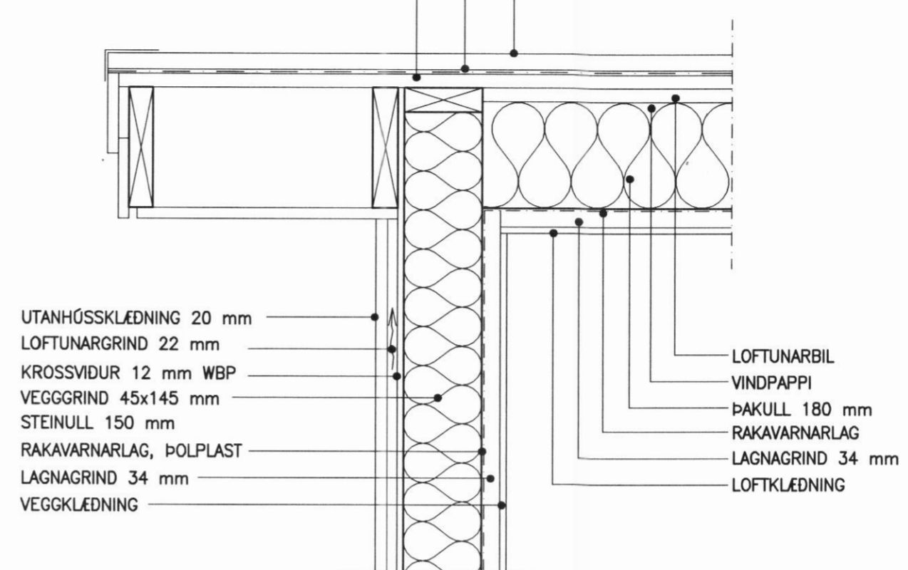
FRÁGANGUR VIÐ ÚTVEGG OG ÞAK/GAFL 1:10
