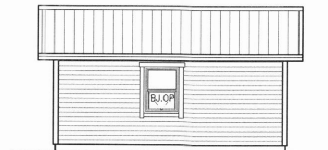
ÚTLIT NORDURHLIÐ
