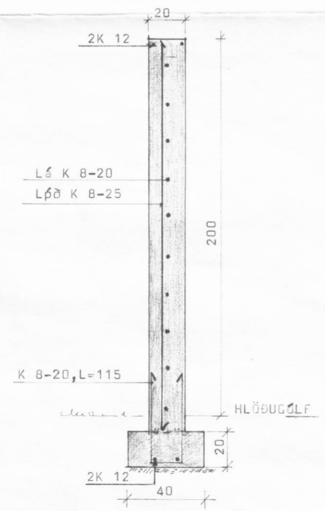
SNID Í GAFL A-A
