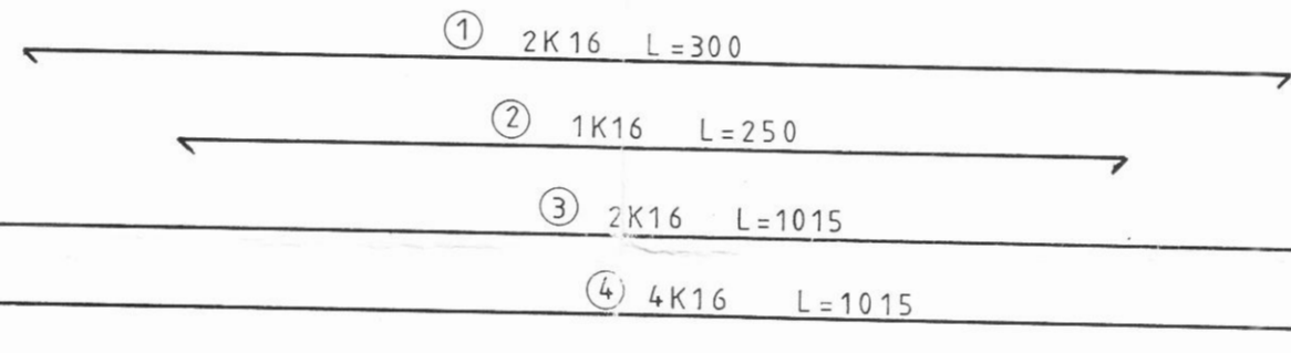
Biti B 3 M=1:20
