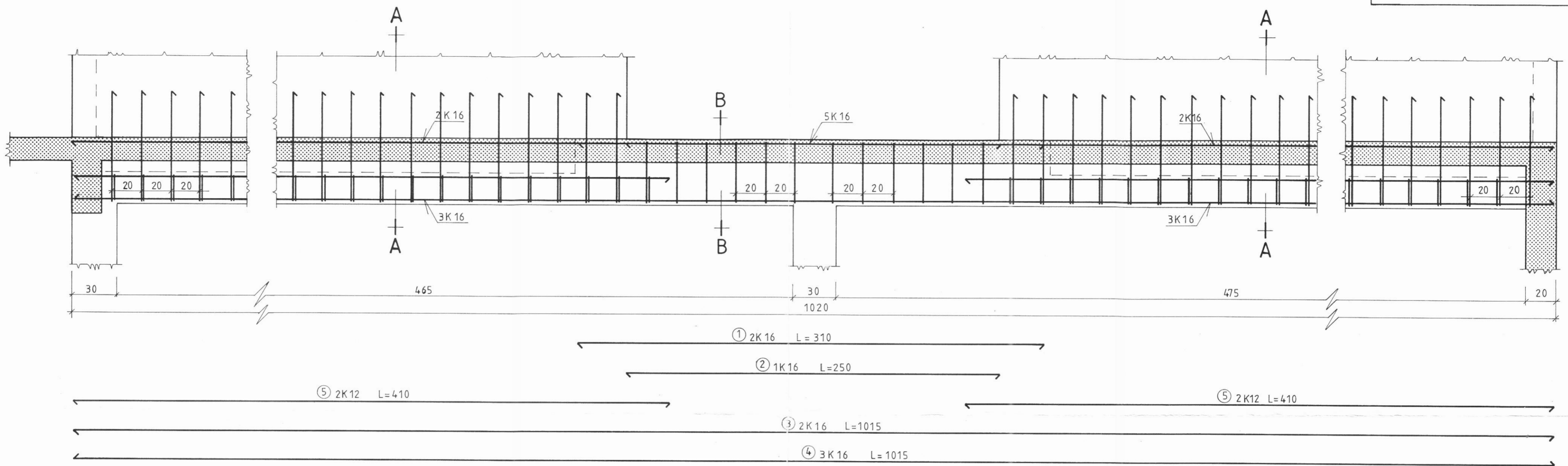
Biti B 2 M=1:20
