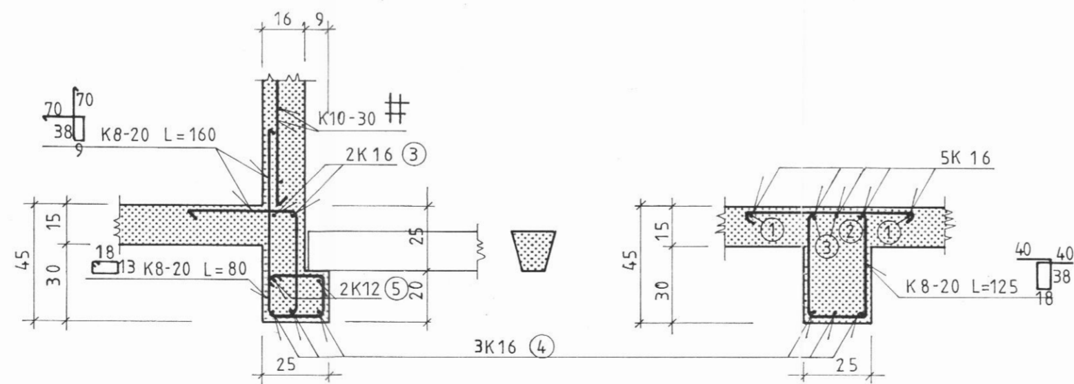
Snið A-A M=1:20
