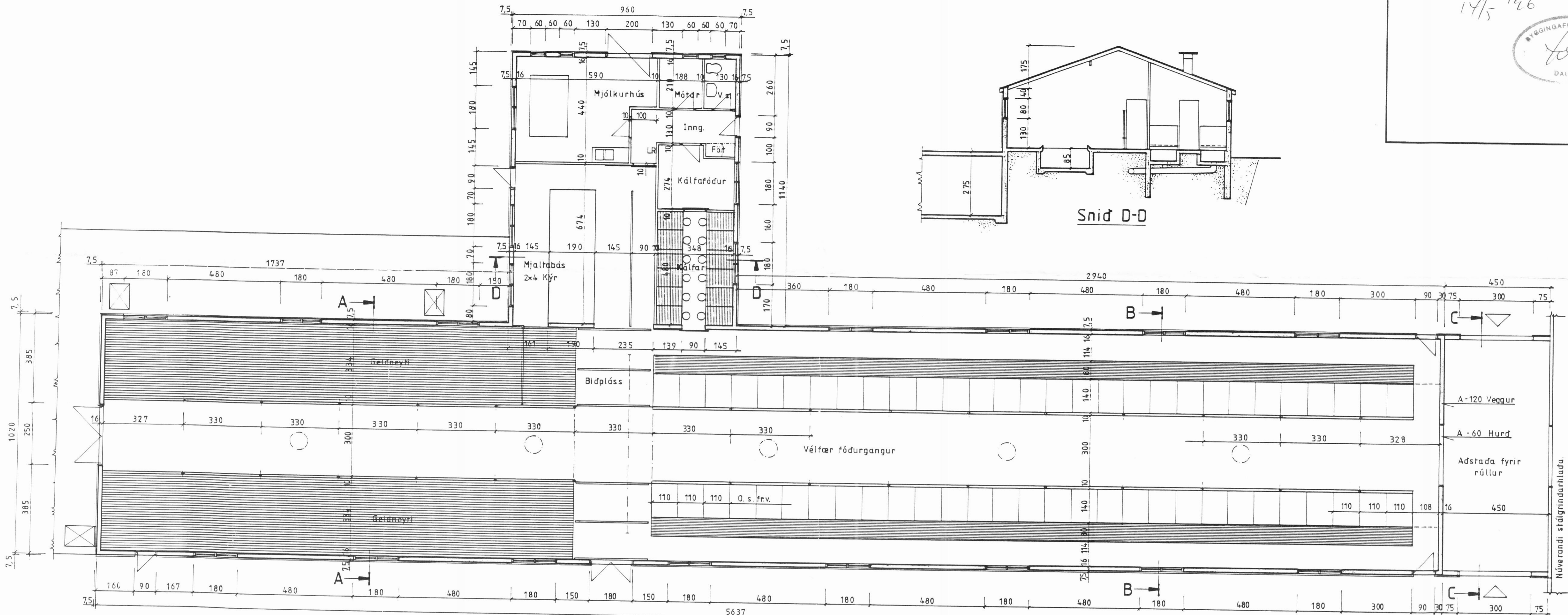
Grunnmynd
