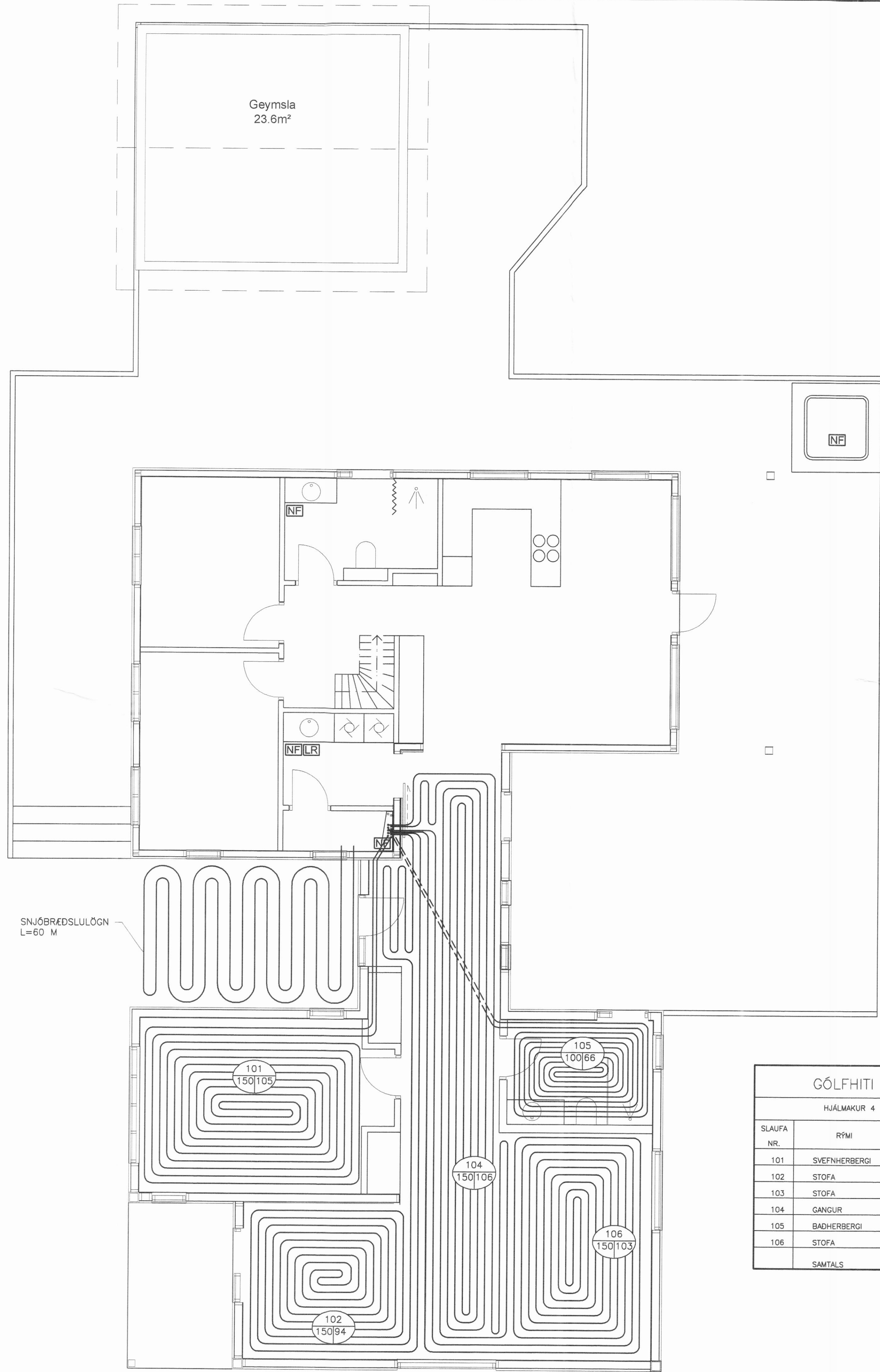
GRUNNMYND. 1:50
