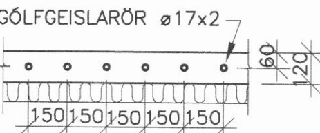
SNID Í GÓLFGEISLALÖGN. 1:20
