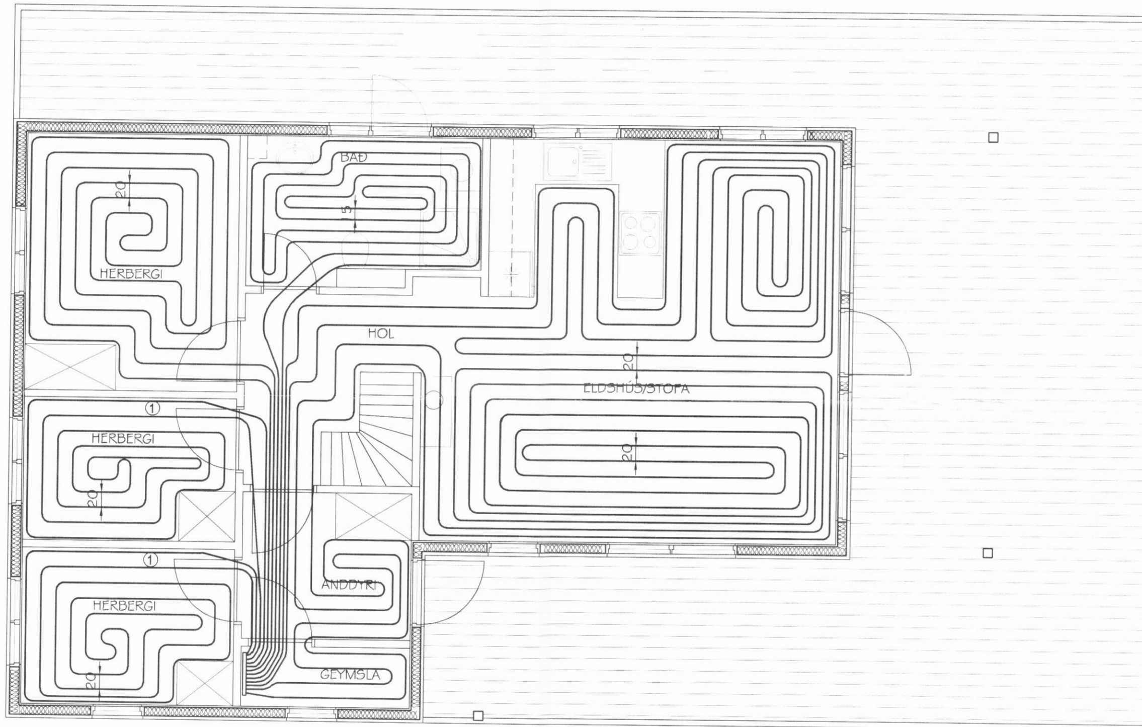
GÓLFHITALGNIR - GRUNNMYND MKV.1 :50
