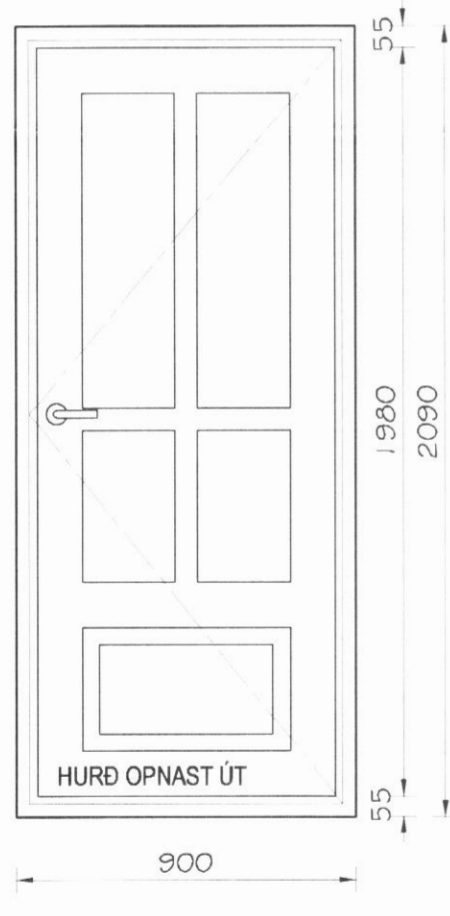
H01 2 STK
