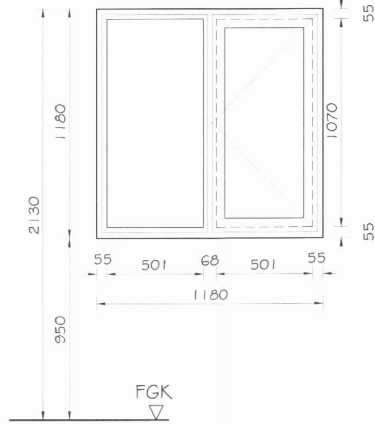
G02 1 STK
