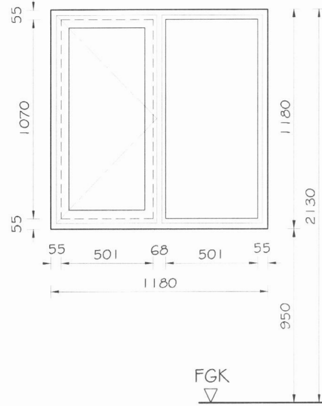
G01 5 STK
