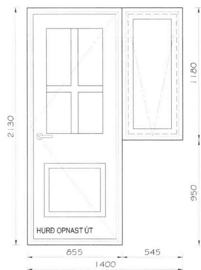
H02 1 STK
