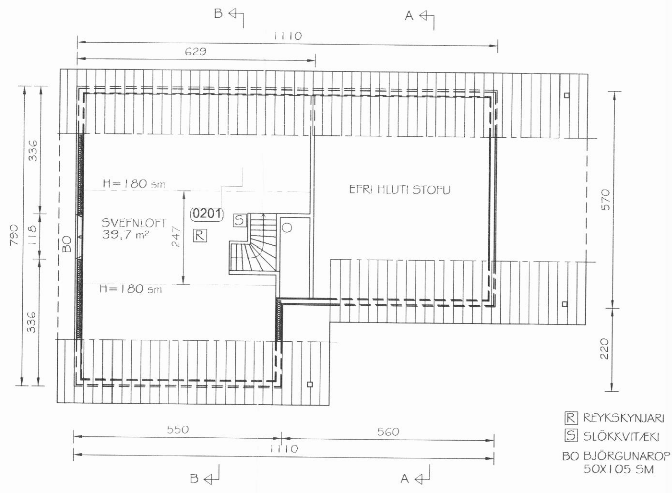
GRUNNMYND SVEFNLOFTS MKV. 1:100
