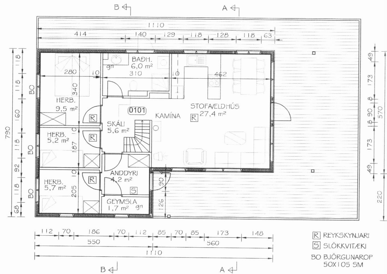
GRUNNMYND MKV. 1:100
