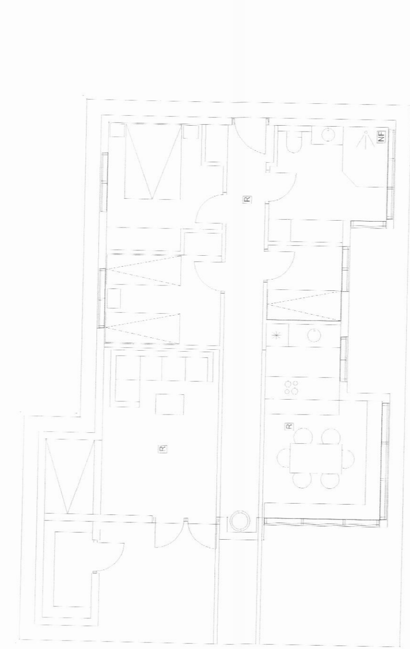
GRUNNMYND 1:100
