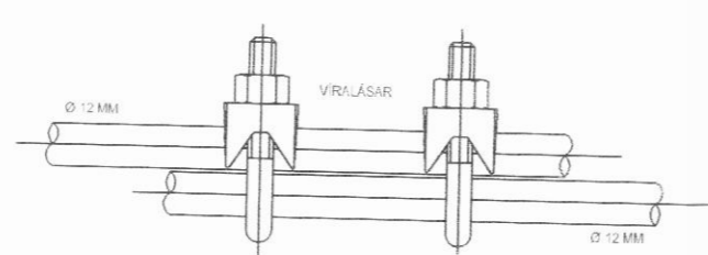
SETJA SKAL TVO VIRALÁSA Á HVER SAMSKEYTI
