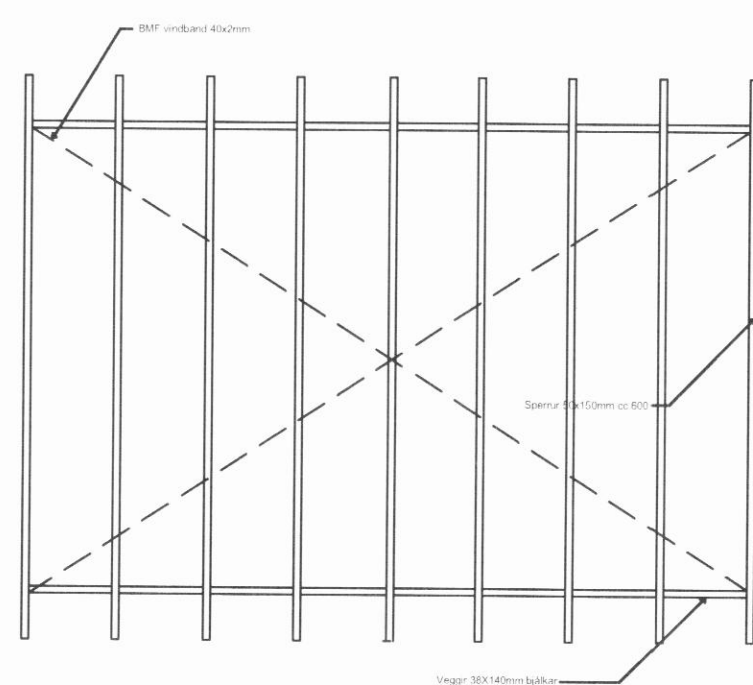
Pakviðir grunnmynd Mhl 02 1:50
