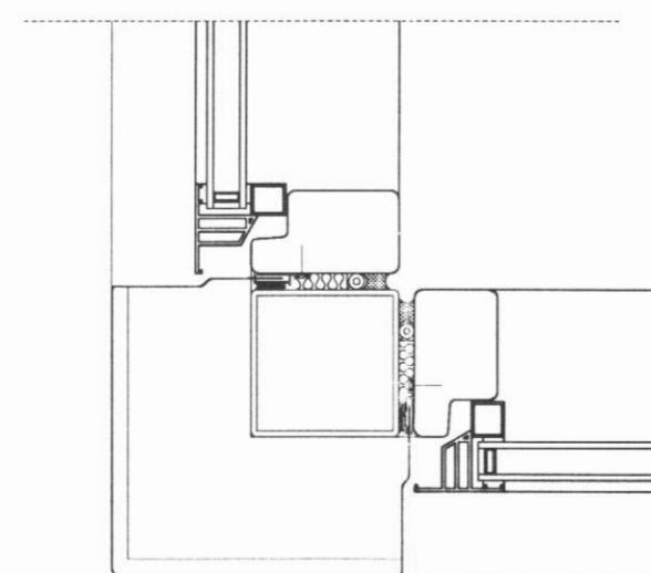
C Hornfrágangur glugga 200 Lárétt deili
