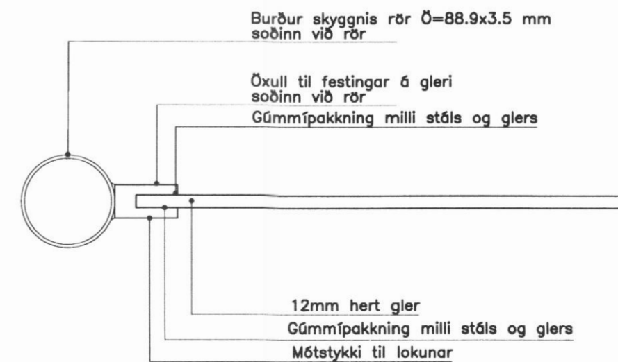
D Glerlokun framan við inngang 200 Lárétt deili
