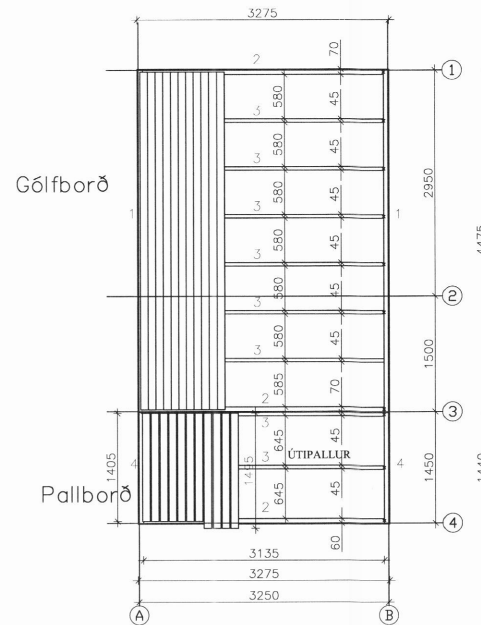
Grunnmynd gólfborð
