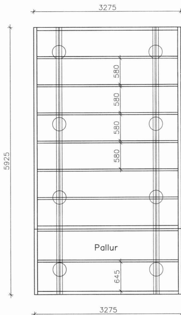
Grunnmynd dregarar
