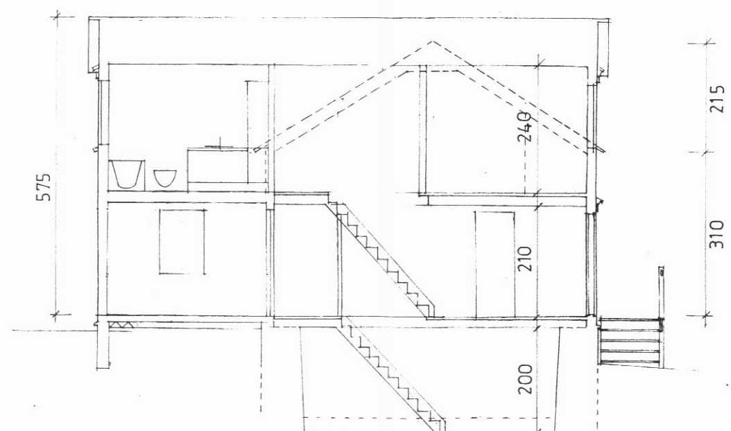
sneiðing 1:100
