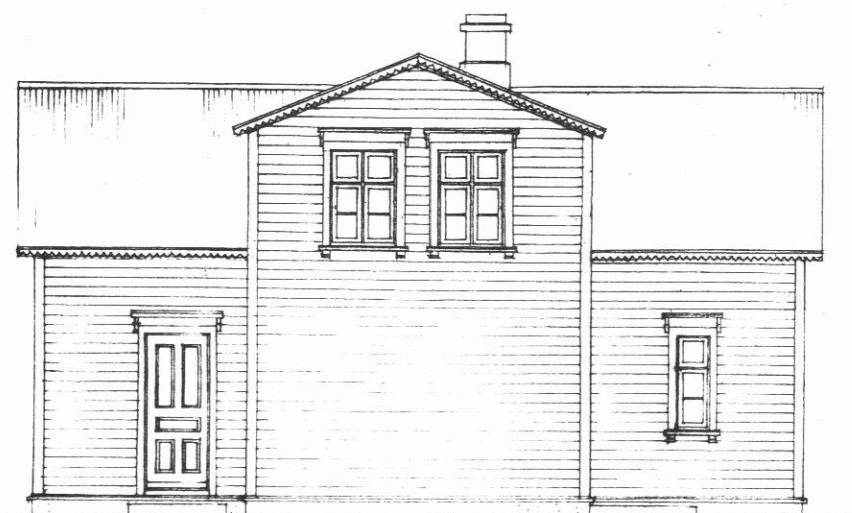
útlit austur 1:100
