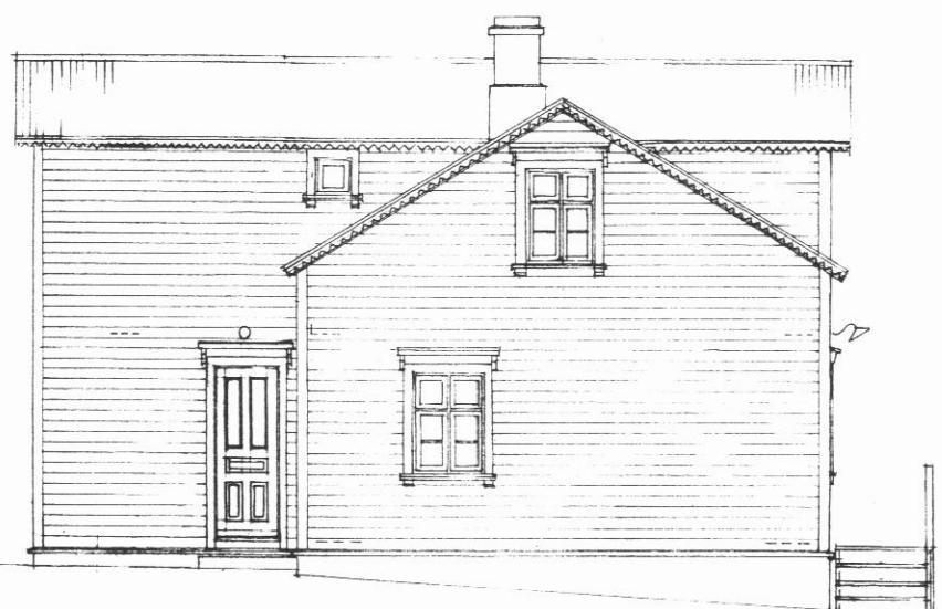
útlit norður 1:100
