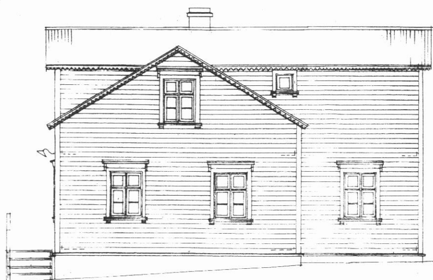
útlit suður 1:100
