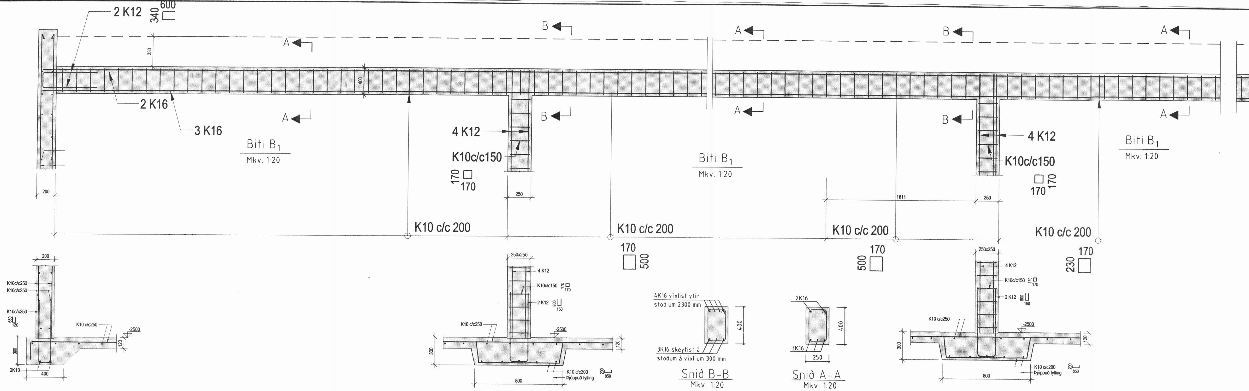
Snið C-C (Fyrri hluti)
