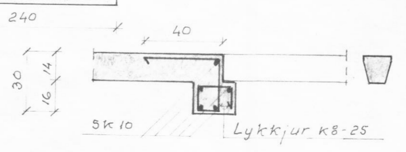
Snið B-B
