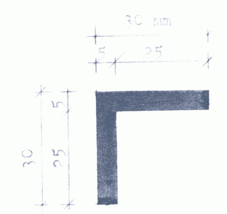
snillingur í burðarvinkil, m.kv. 1:1 vinklarnir smíðast úr stáli og hálðast með rilsan
