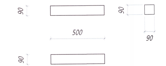
Nr. 137 HB Hurðabiti Límré: 90*90, L=500 mm Samtals: 4 stk.
