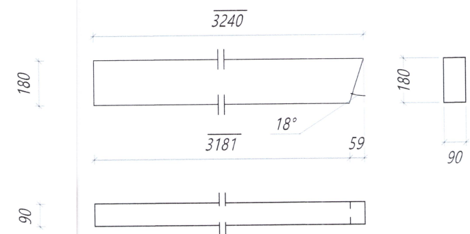
Nr. 123 HS Hurðastoð Límré: 90*180, L=3240 mm Samtals: 2 stk.
