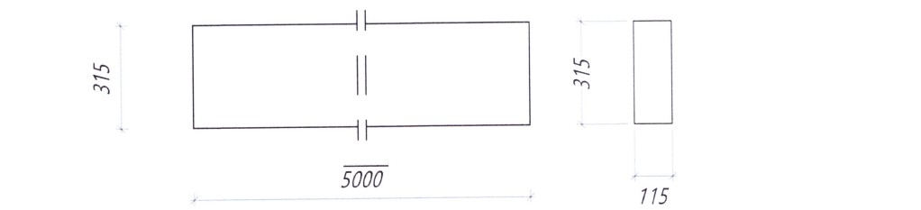
Nr. 131 HB Hurðabiti Límré: 115*315, L=5000 mm Samtals: 1 stk.
