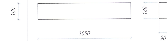
Nr. 126 HB Hurðabiti Límré: 90*180, L=1050 mm Samtals: 1 stk.
