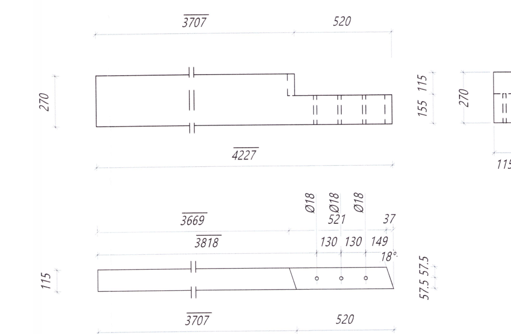
Nr. 135 GS Gafstoð Límré: 115*270, L=4227 mm Samtals: 1 stk.
