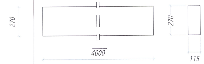
Nr. 124 HB Hurðabiti Límré: 115*270, L=4000 mm Samtals: 1 stk.
