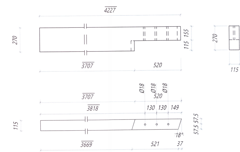
Nr. 136 GS Gafstoð Límré: 115*270, L=4227 mm Samtals: 1 stk.
