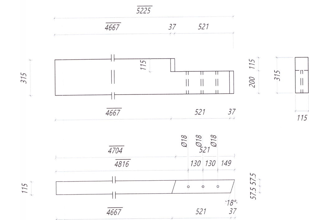
Nr. 134 GS Gafstoð Límré: 115*315, L=5225 mm Samtals: 1 stk.
