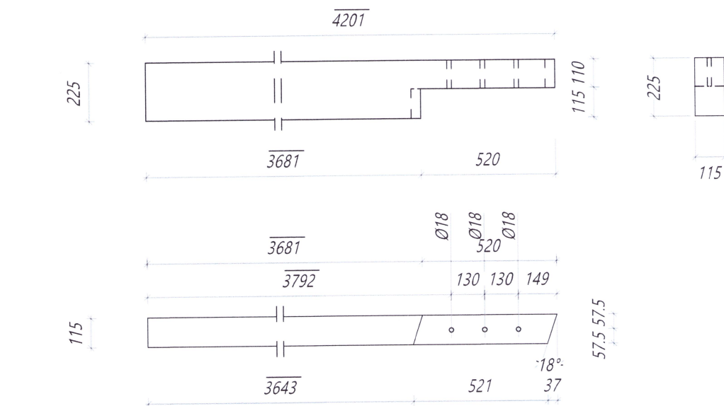
Nr. 130 GS Gafstoð Límré: 115*225, L=4201 mm Samtals: 1 stk.
