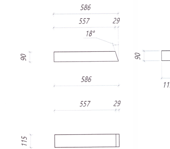
Nr. 138 HB Hurðabiti Límré: 115*90, L=586 mm Samtals: 1 stk.
