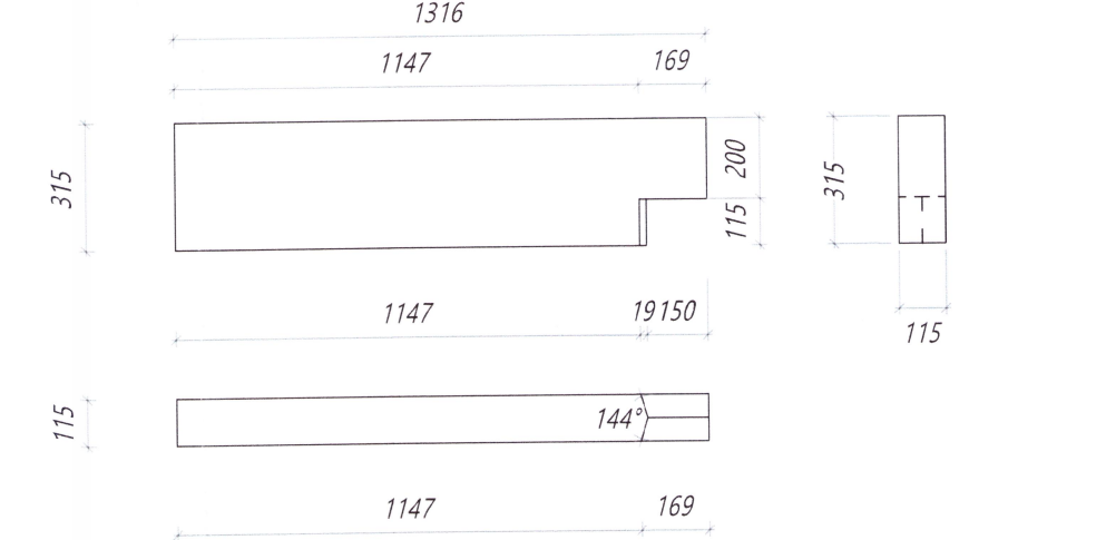
Nr. 132 Hurðabiti Límré: 115*315, L=1316 mm Samtals: 1 stk.
