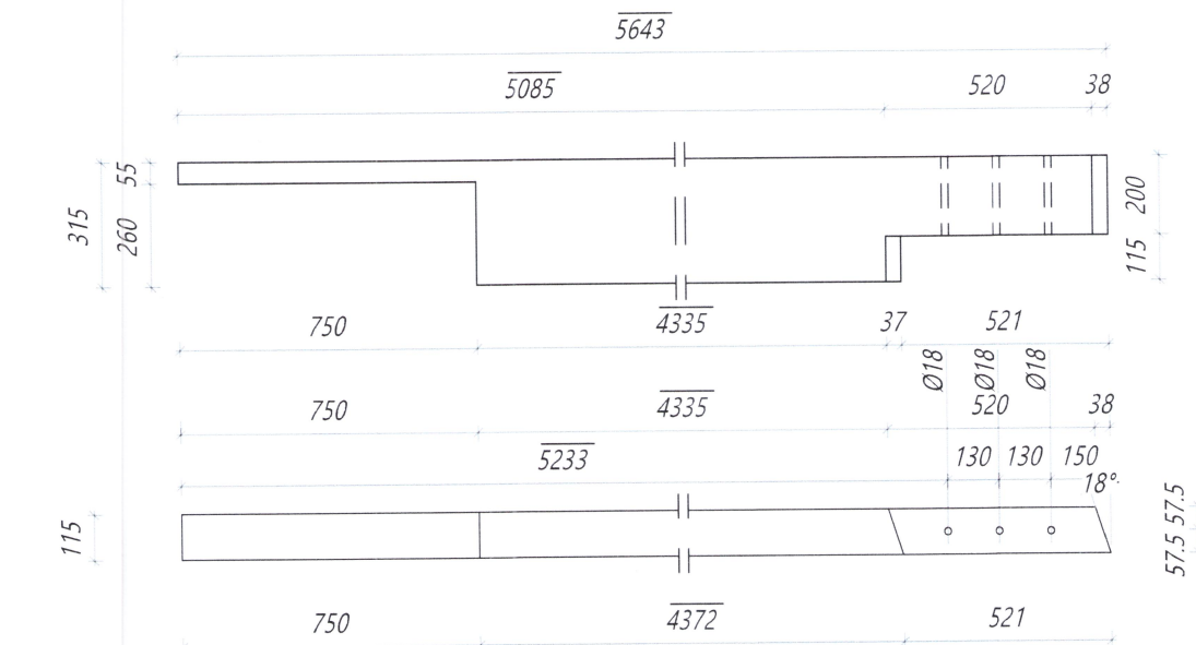
Nr. 127 HS Hurðastoð Límré: 115*315, L=5643 mm Samtals: 1 stk.
