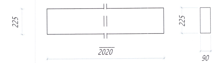
Nr. 125 HB Hurðabiti Límré: 90*225, L=2020 mm Samtals: 1 stk.
