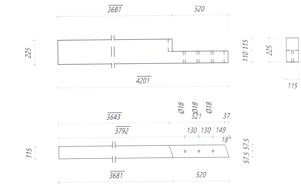
Nr. 129 GS Gafstoð Límré: 115*225, L=4201 mm Samtals: 1 stk.
