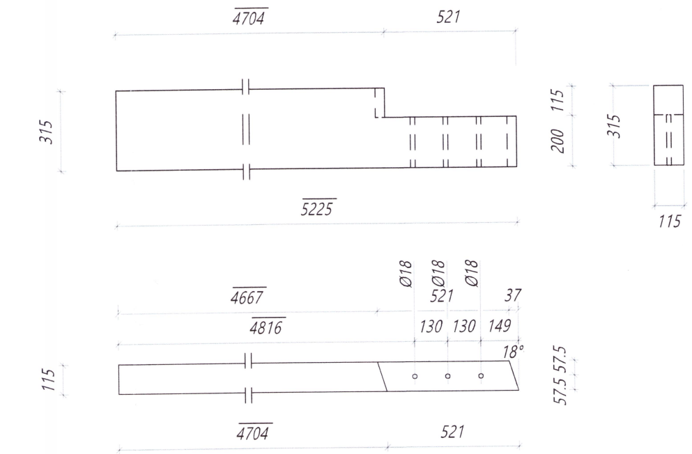
Nr. 133 GS Gafstoð Límré: 115*315, L=5225 mm Samtals: 1 stk.
