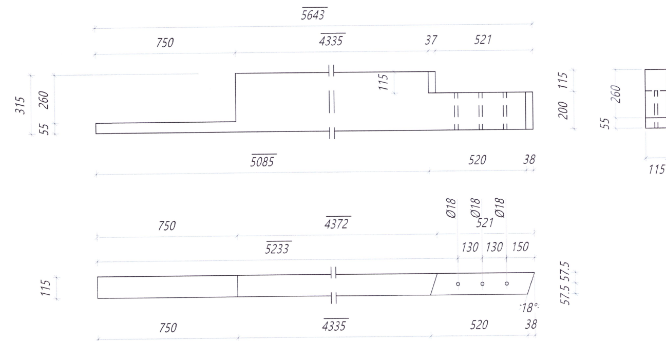
Nr. 128 HS Hurðastoð Límré: 115*315, L=5643 mm Samtals: 1 stk.
