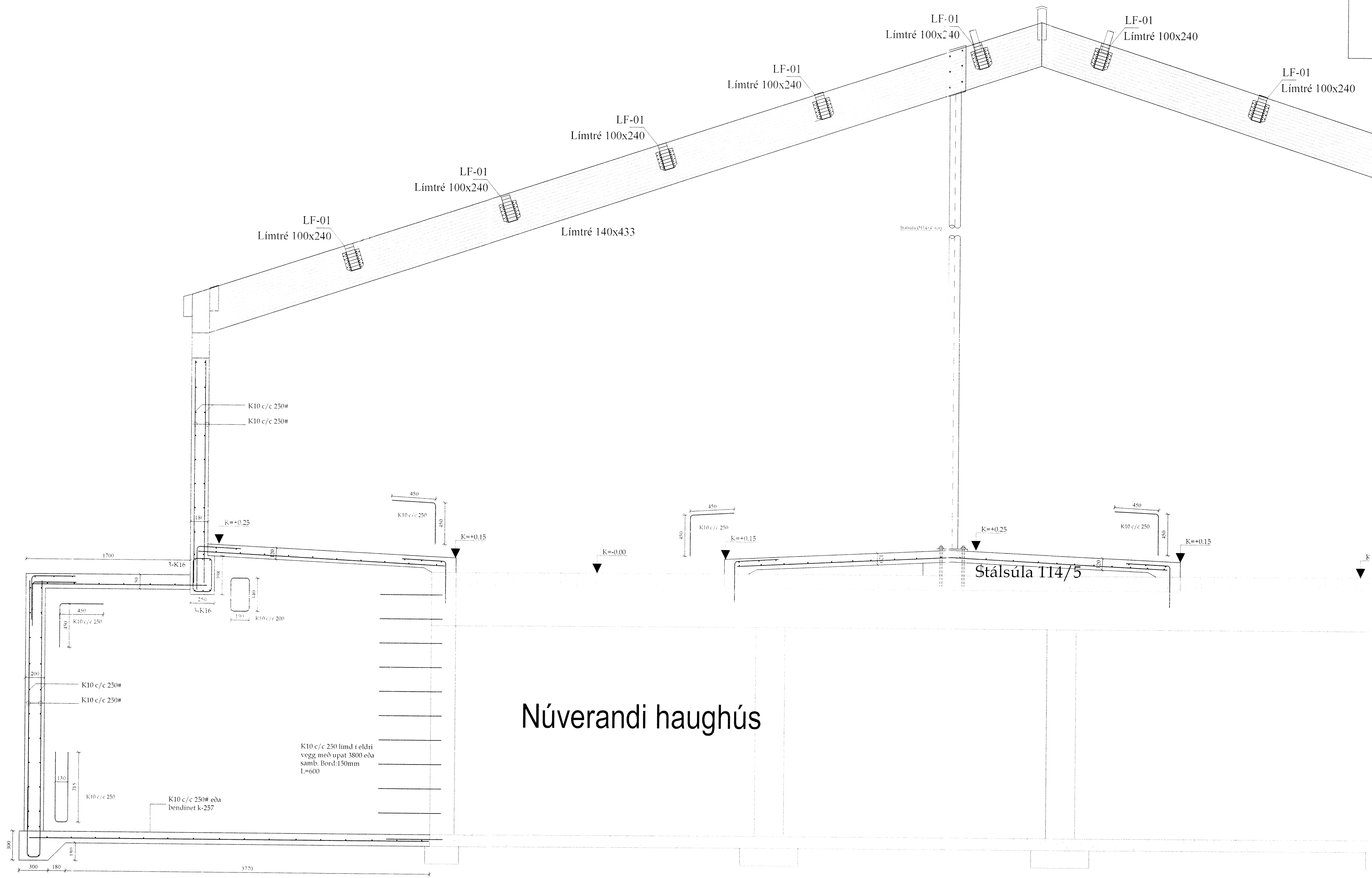
Þversnið B-B mk. 1:20
