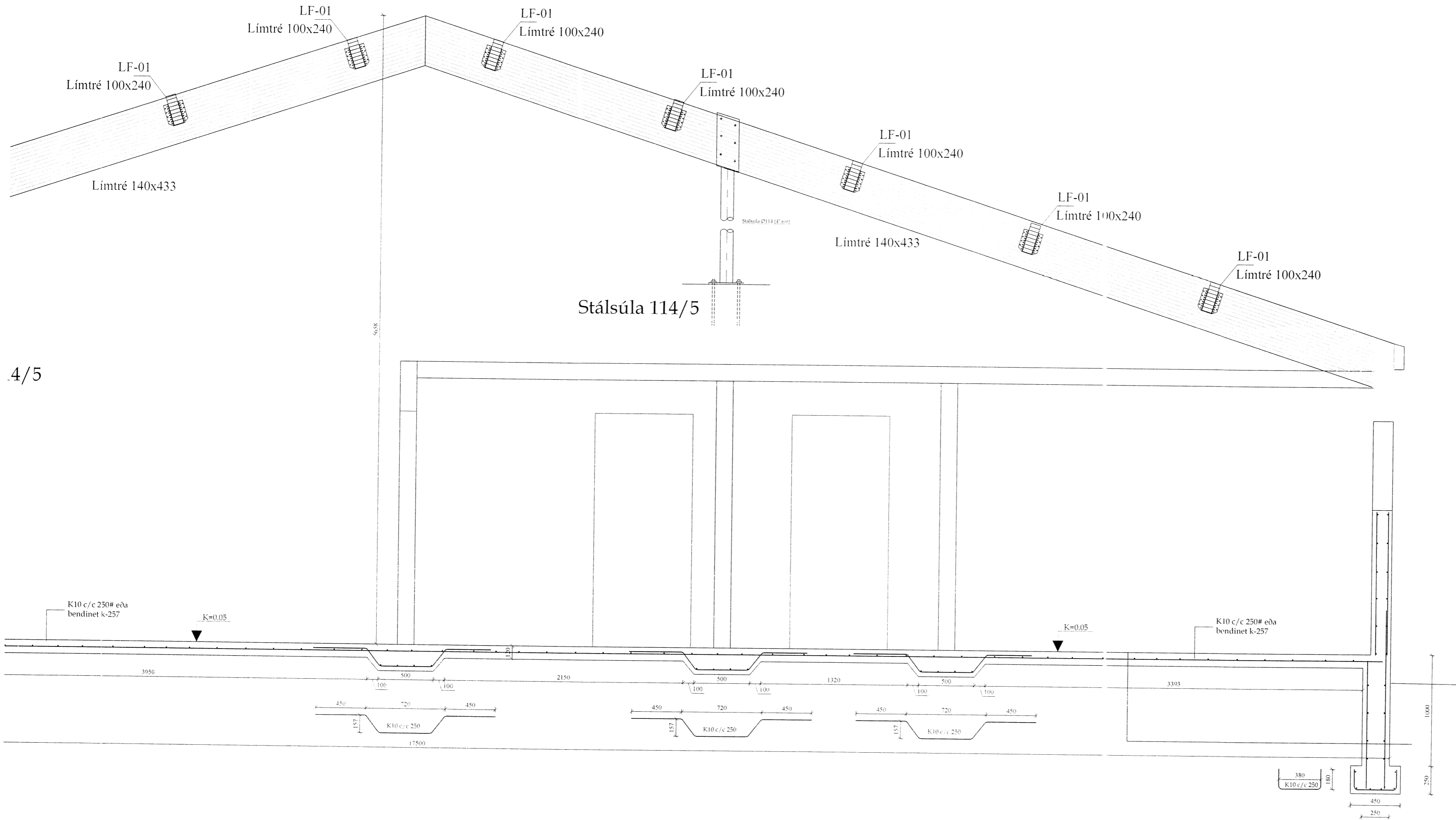
Þversnið A-A hluti 2 mk. 1:20
